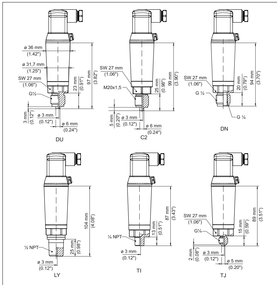
插图. 29: VEGABAR 29, 螺纹, 非正面齐平式
