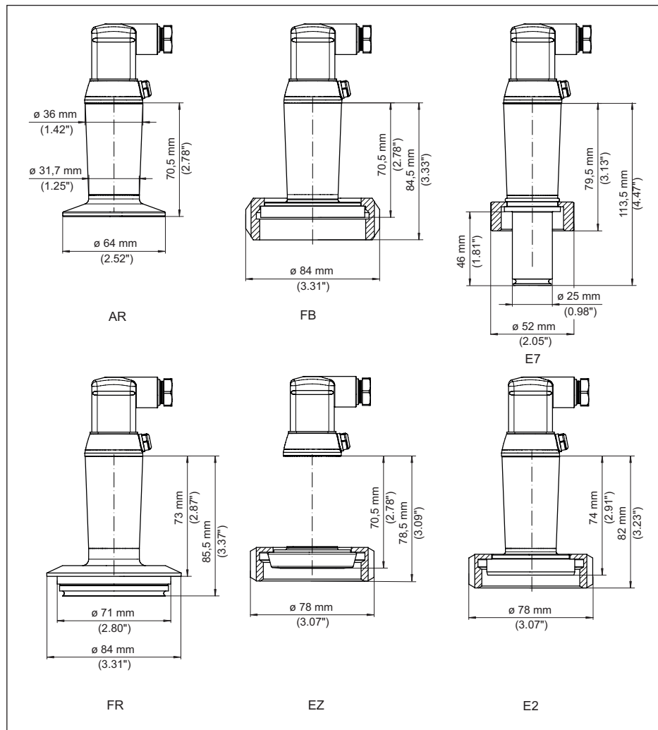
插图. 32: VEGABAR 29, 卫生型接口
