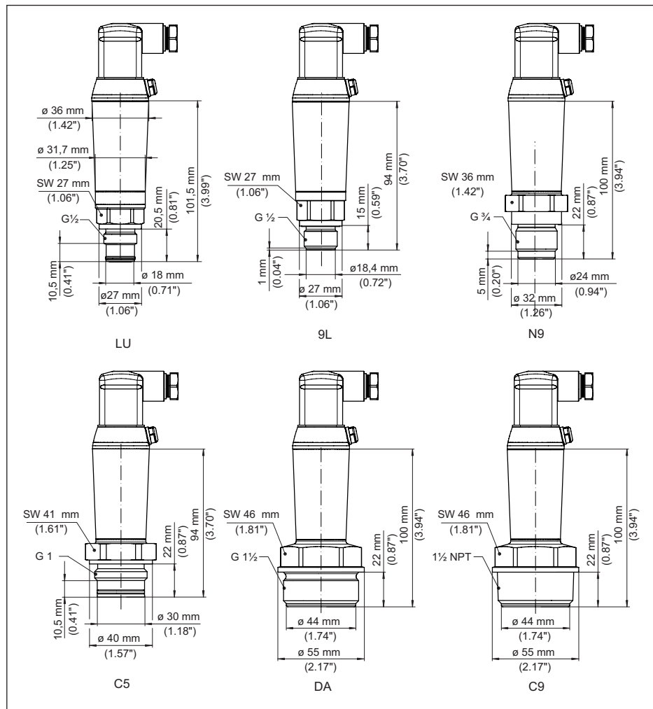
插图. 30: VEGABAR 29, 螺纹接头正面齐平式
