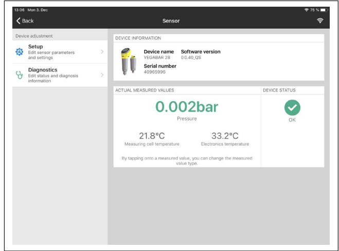
插图. 20: App 视图举例 - 调试 测量值
