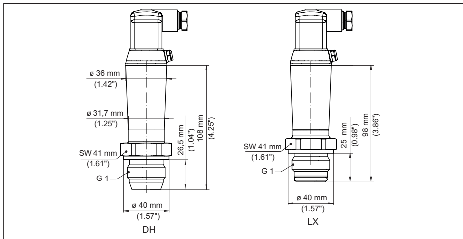
插图. 31: VEGABAR 29, 锥/管接口
