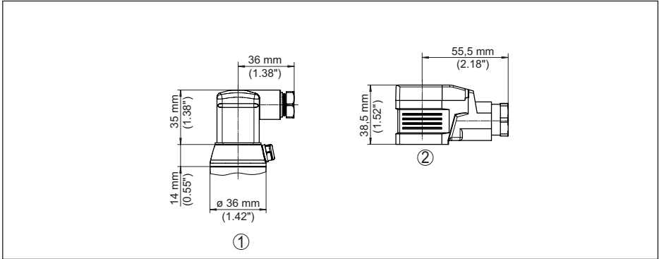
插图. 28: VEGABAR 29 的连接技术
