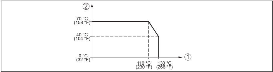
插图. 26: VEGABAR 29 的温度降额
