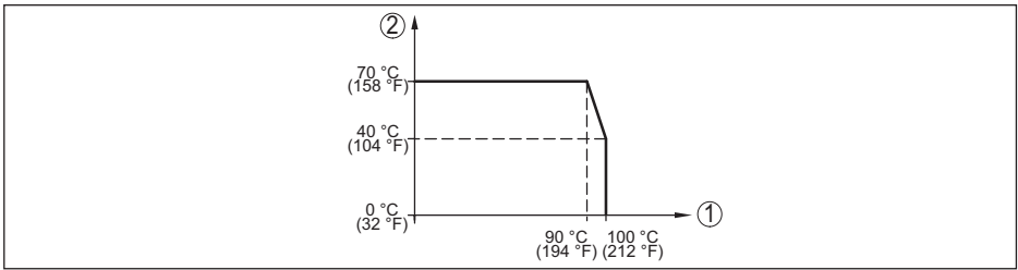
插图. 27: 温度降额 VEGABAR 29, 当蓝牙通信激活时
