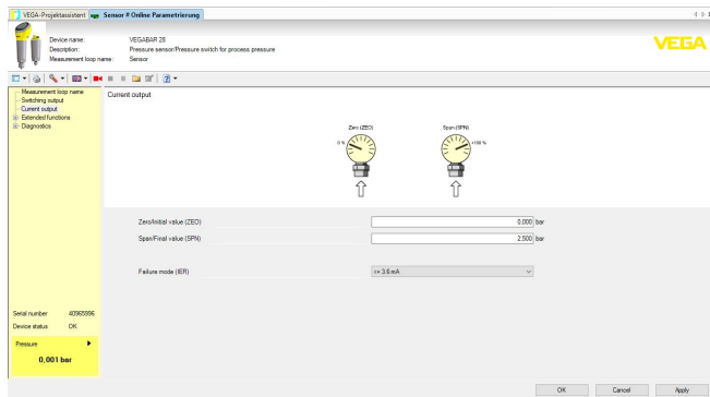
插图. 22: DTM 视图举例 - 调整电流输出
