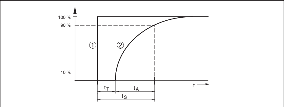
插图 24: 出现过程值跳跃式变化时电流输出的表现。t T : 停滞时间; t A : 上升时间; t S : 跳跃式响应时间
