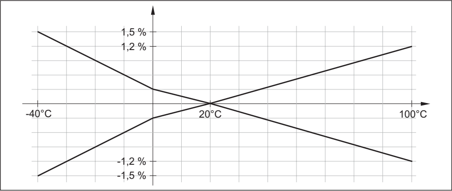
插图. 25: 在 TD 1 : 1 时的温度误差
