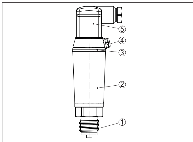
插图. 1: VEGABAR 29的部件
