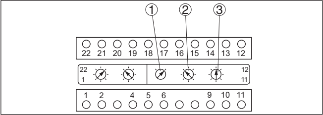
插图. 18: 地址选择开关
