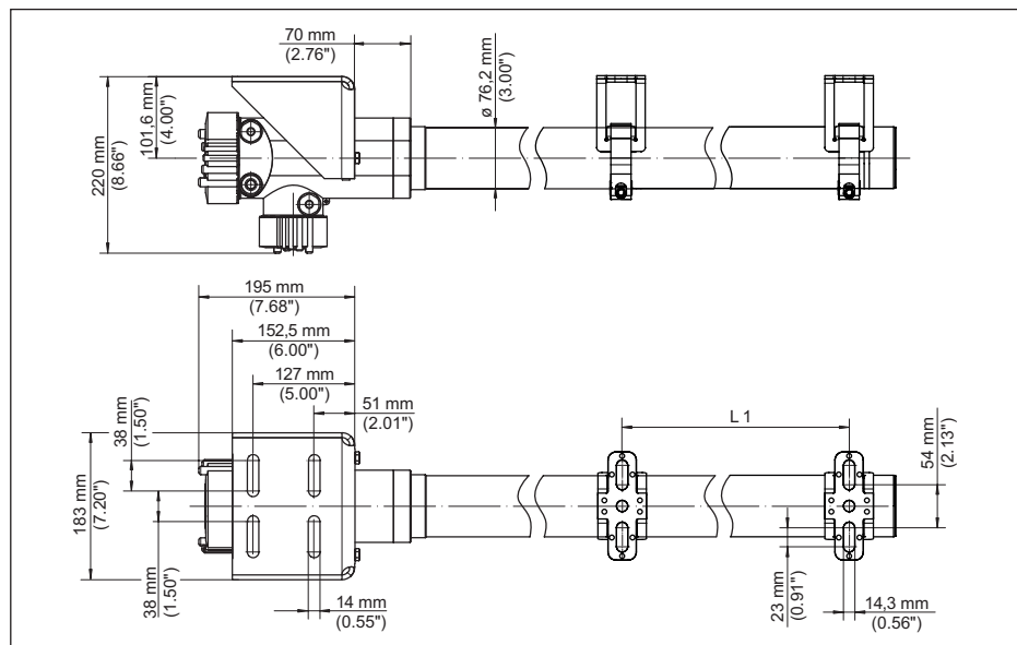
插图. 31: SOLITRAC 31 带随附的安装配件
