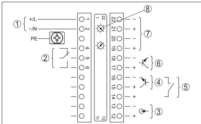
插图. 15: 在带有自安全电流输出出口的仪表上的电子部件和接线腔 (防爆 (Ex d))
