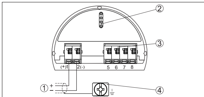
插图. 12: 在带有自安全电流输出出口的仪表上的操作和接线腔 (防爆 (Ex ia))
