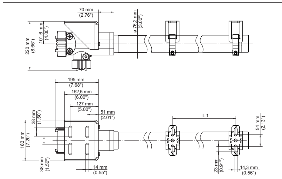
插图. 28: SOLITRAC 31 带随附的安装配件
