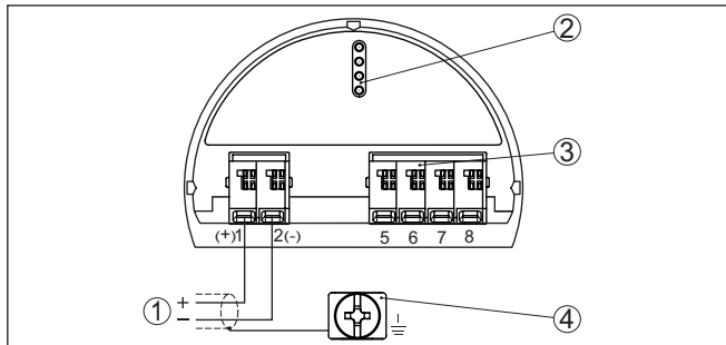
插图. 16: 在带有自安全电流输出出口的仪表上的操作和接线腔 (防爆 (Ex ia))
