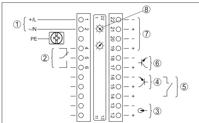
插图. 11: 在带有自安全电流输出出口的仪表上的电子部件和接线腔 (防爆 Ex d)
