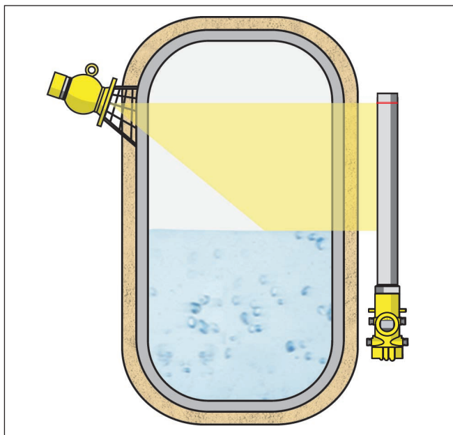
插图. 7: 在一个带热绝缘的加热容器上测量物位
