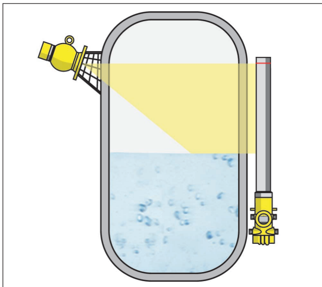
插图. 4: 在一个储罐上测量物位
