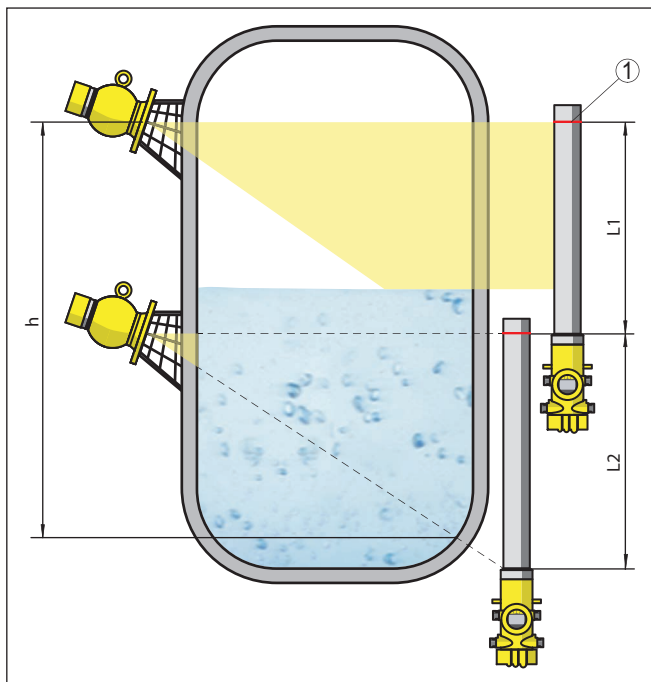
插图. 6: 安装位置 - 串联排列
