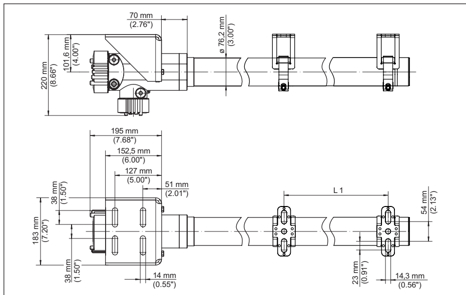
插图. 27: SOLITRAC 31 带随附的安装配件
