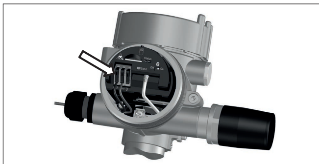
插图. 2: 接线步骤 4 和 5
