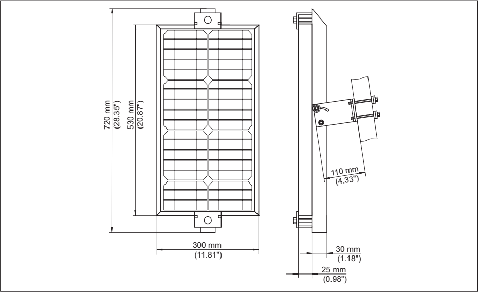
插图. 14: PLICSMOBILE S81 的尺寸
