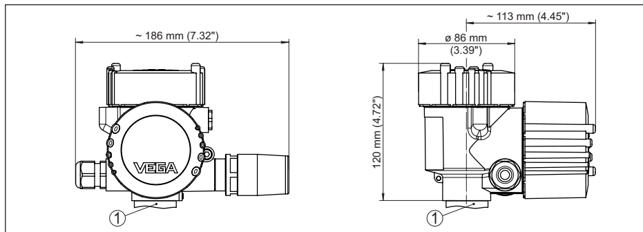
插图. 12: 带有不锈钢/铝壳体的 PLICSMOBILE 81 的尺寸
