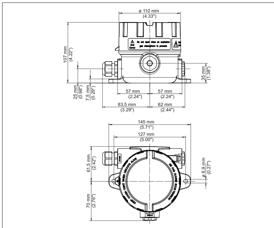
插图. 13: 带有铝壳体的 PLICSMOBILE B81 的尺寸
