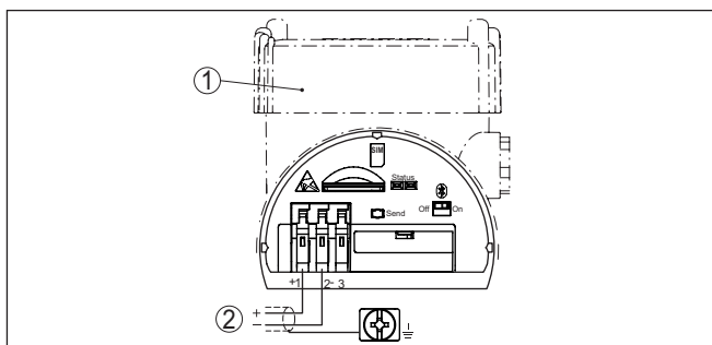
插图. 3: PLICSMOBILE 81 的供电装置的连接
