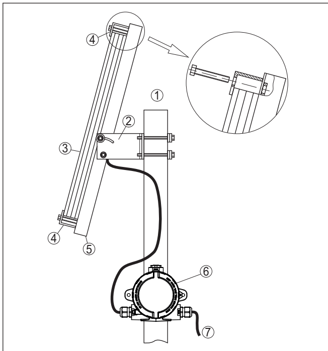
插图. 5: 将 PLICSMOBILE 通过管件式安装与太阳能电池组件相连
