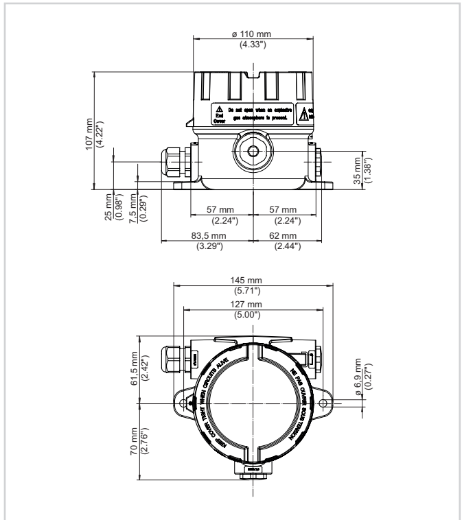
帶有鋁殼體的 PLICSMOBILE B81 的尺寸
