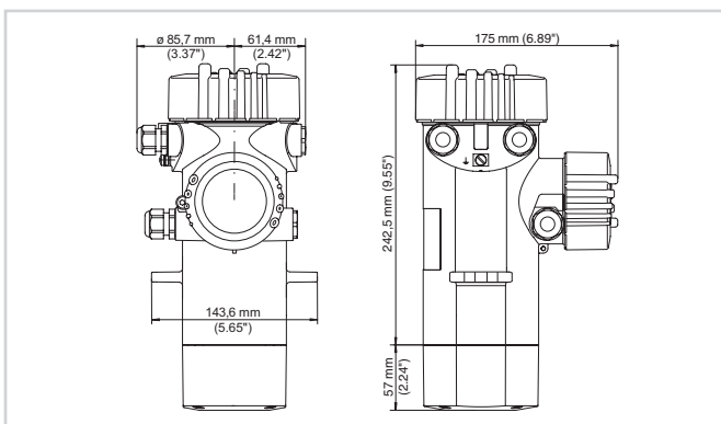
MINITRAC 31 的尺寸
