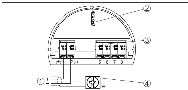
插图. 14: 在带有本安型信号输出出口的仪表上的操作和接线腔 (防爆 Ex ia) 型)
