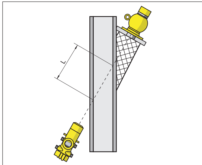
插图. 22: 斜向安装时适用管件的辐照长度
