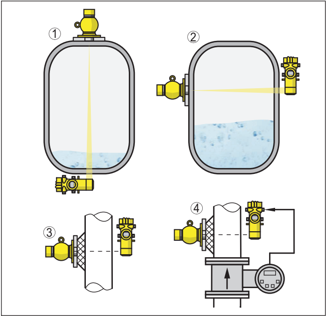
插图. 2: MINITRAC 31 - 可能的用途
