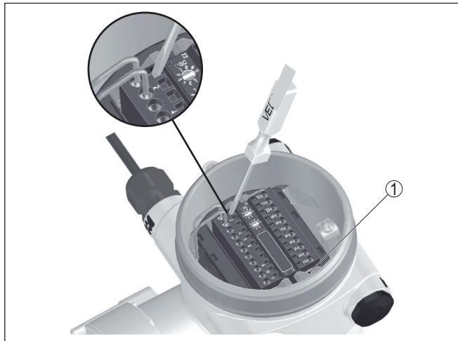
插图. 10: 接线步骤 4 和 5
