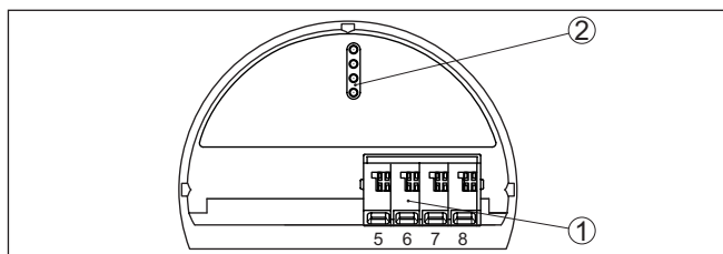
插图. 12: 非防爆型仪表和带有非本安型信号输出口的仪表上的操作和接线腔
