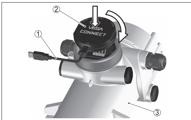
插图. 23: 通过接口适配器将电脑直接与仪表相连
