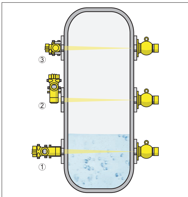
插图. 8: 安装位置 - 极限物位测量
