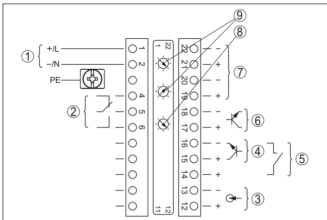
插图. 17: 在带有本安型信号输出出口的仪表上的电子部件和接线腔 (防爆 (Ex d) 型)
