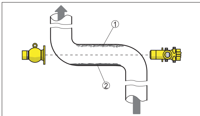
插图. 5: 安装在一根水平管道上
