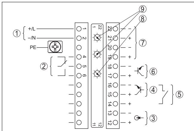
插图. 13: 在带有本安型信号输出出口的仪表上的电子部件和接线腔 (防爆 Ex d) 型)
