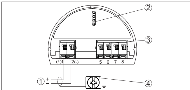
插图. 18: 在带有本安型信号输出出口的仪表上的操作和接线腔 (防爆 (Ex ia) 型)
