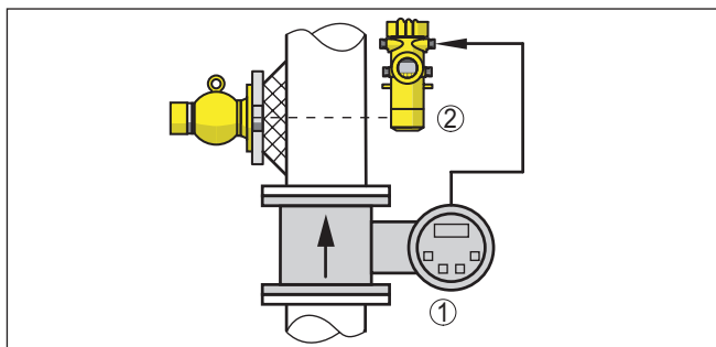
插图. 7: 测量质量流量
