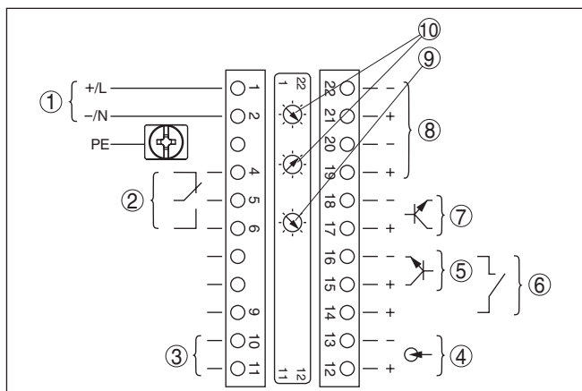
插图. 11: 非防爆型仪表和带有非本安型信号输出口的仪表上的电子部件和接线腔
