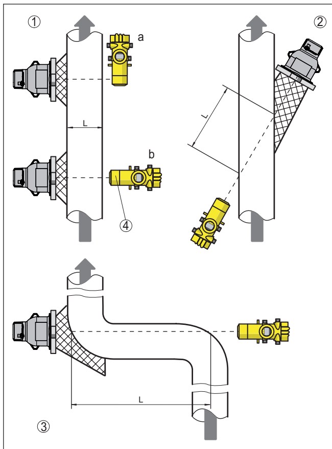
插图. 6: 安装变种 - 密度测量或浓度测量
