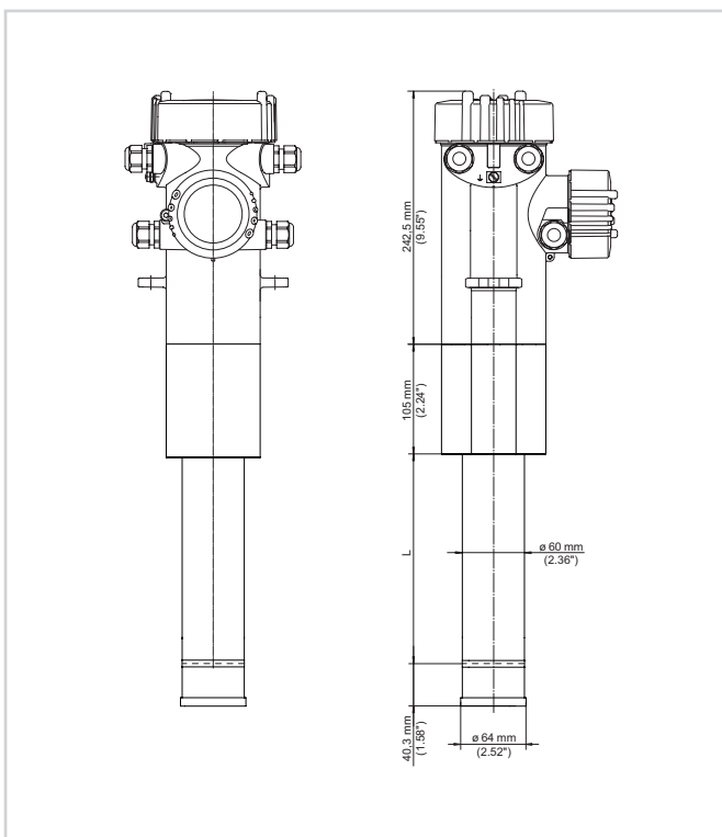
FIBERTRAC 32 的尺寸
