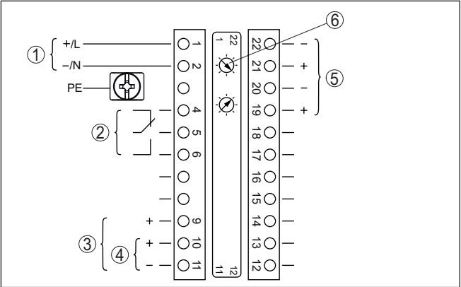
插图. 12: 非防爆仪表和带有非自安全电流输出出口的仪表上的电子部件和接线腔
