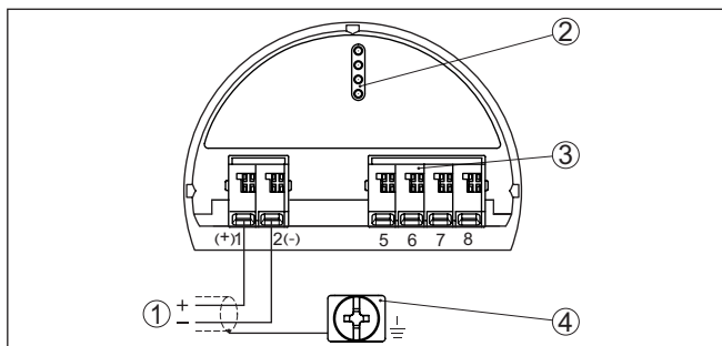
插图. 11: 在带有自安全电流输出出口的仪表上的操作和接线腔 (防爆 (Ex ia))
