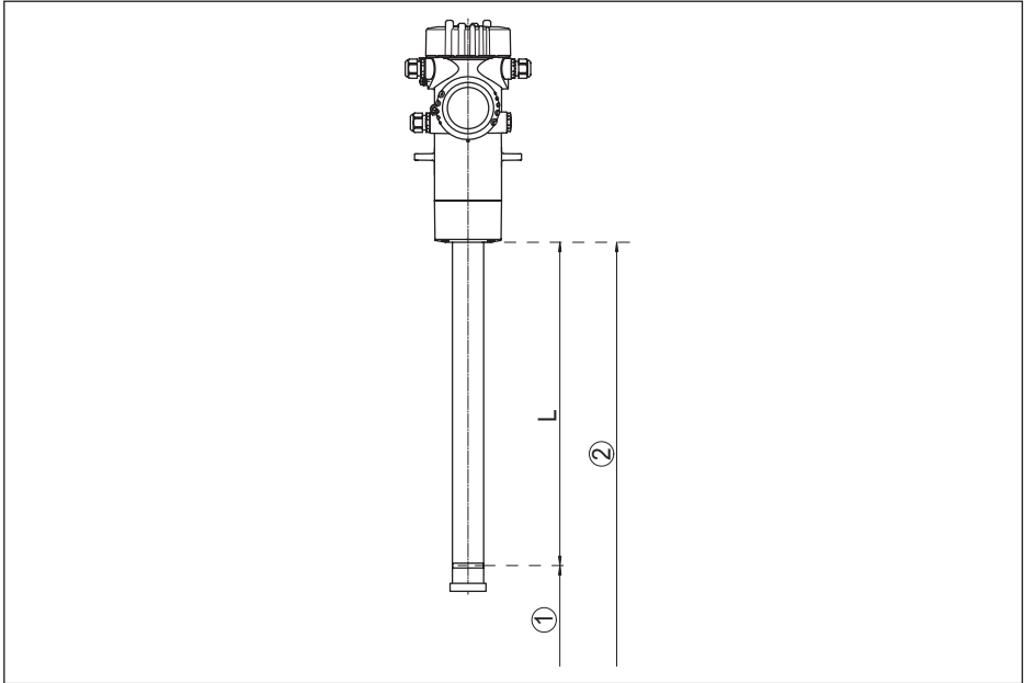
插图. 26: 有关输入值的信息 1 最小物位 (红色的标记线) 2 最大物位 L 测量范围 (仪表的订购长度)
