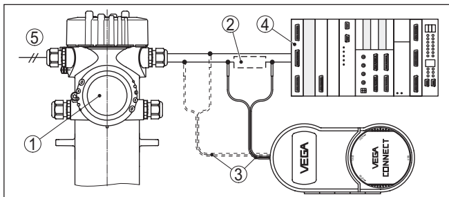
插图. 22: 通过 HART 将电脑与信号线路相连
