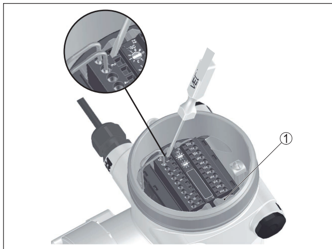
插图. 7: 接线步骤 4 和 5
