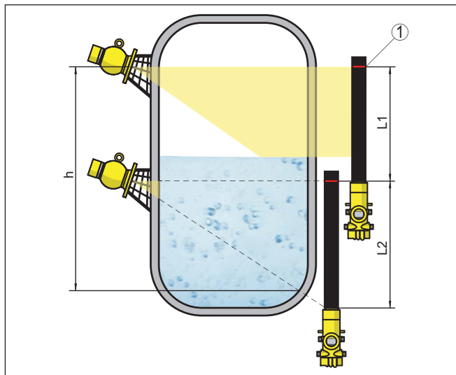
插图. 5: 安装位置 - 串联排列
