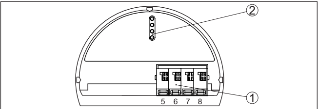
插图. 13: 非防爆仪表和带有非自安全电流输出出口的仪表上的操作和接线腔
