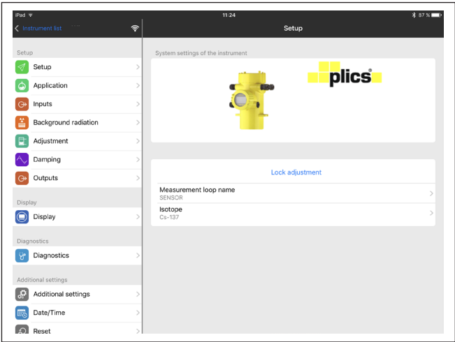
插图. 20: App 视图举例 - 调试 测量值
