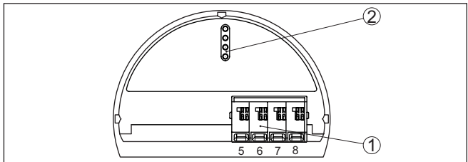
插图. 9: 非防爆仪表和带有非自安全电流输出出口的仪表上的操作和接线腔
