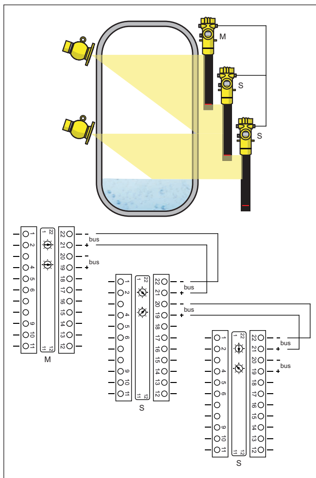
插图. 16: 在串联多个仪表时的电子部件和接线腔。
