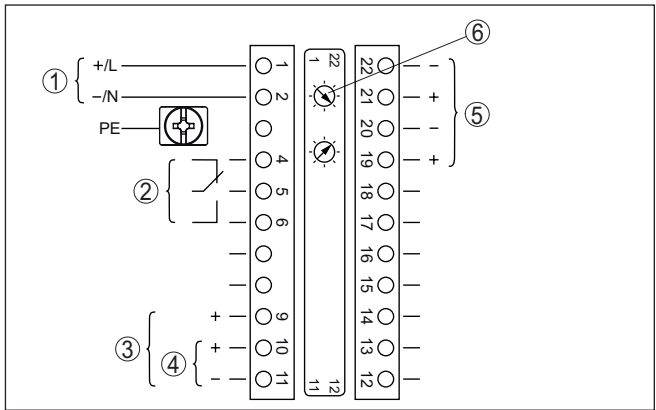
插图. 8: 非防爆仪表和带有非自安全电流输出出口的仪表上的电子部件和接线腔
