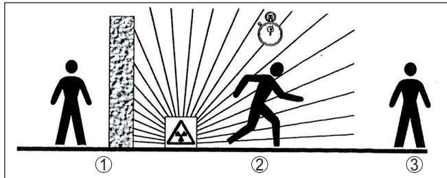
插图 2: 放射性辐射的防护措施
