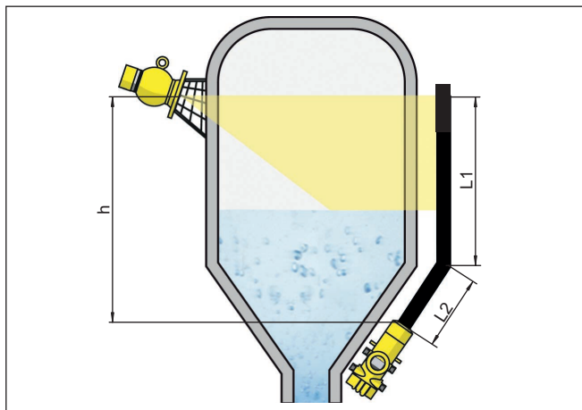
插图. 3: 在一个储罐上测量物位
