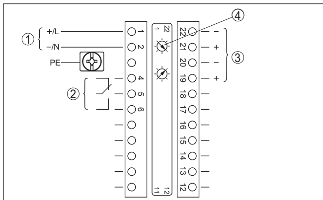
插图. 10: 在带有自安全电流输出出口的仪表上的电子部件和接线腔 (防爆 (Ex d))
