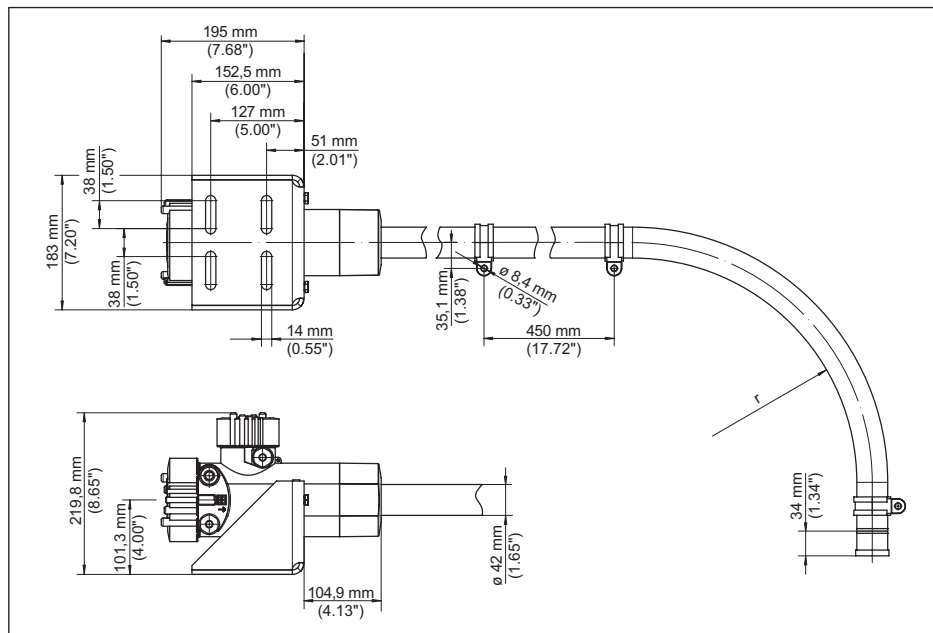
插图. 29: FIBERTRAC 31 带随附的安装配件
