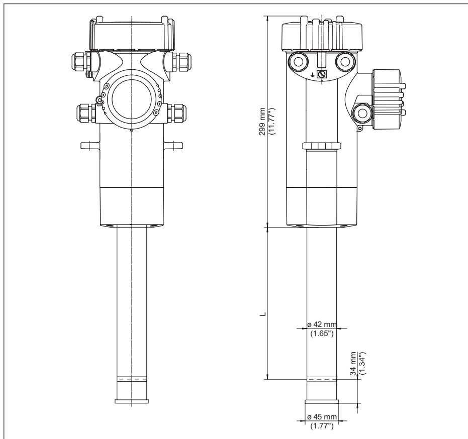
插图. 28: FIBERTRAC 31
