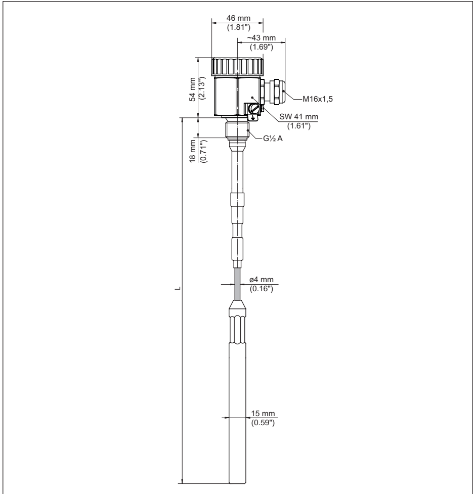
插图. 6: 导电性杆式测量探头EL 9
