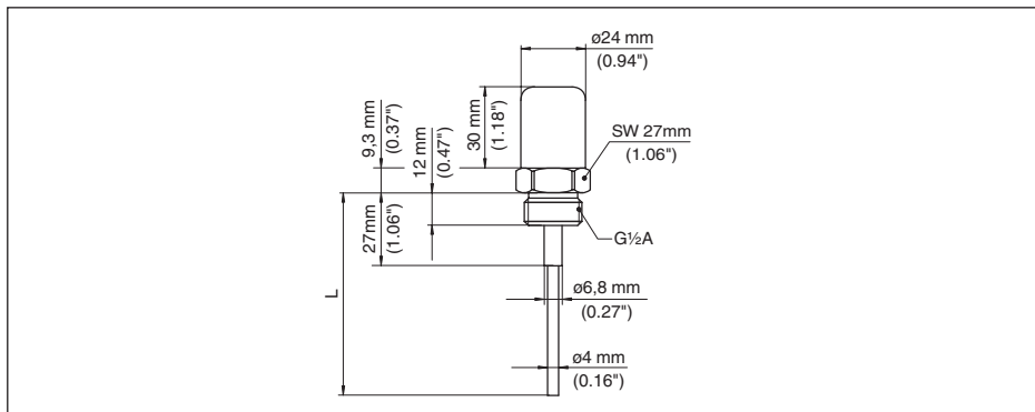
插图 5: 导电性杆式测量探头 EL 8
