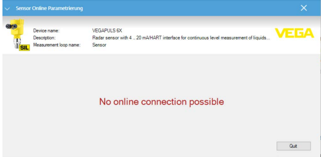
插图. 16: VEGAPULS 6X 在线运行(连接已断开 (非同步)) 时的 DTM 视图
