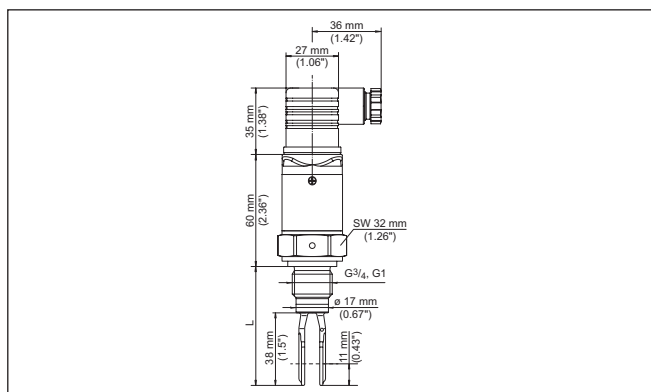
Abb. 32: VEGASWING S51 avec connecteur type électrovanne ISO 4400
