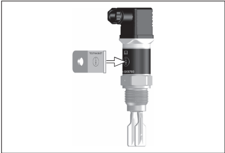
Abb. 41: Simulación de la señal de salida
