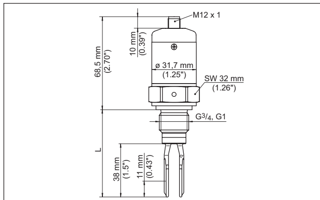
Abb. 9: VEGASWING S51 mit M12 x 1-Steckverbindung
