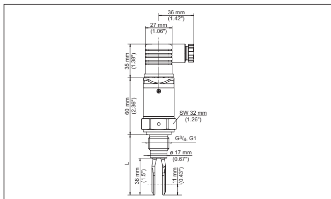
Abb. 43: VEGASWING S51 con enchufe de válvula según DIN 4400
