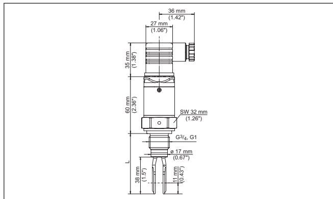
Abb. 10: VEGASWING S51 mit Ventilstecker nach ISO 4400
