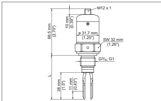
Abb. 42: VEGASWING S51 con conexión de enchufe M12 x 1
