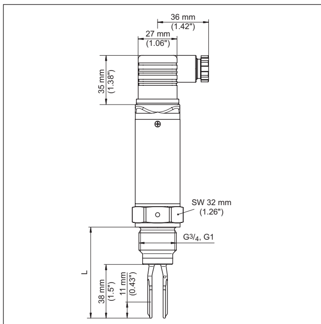
Abb. 11: VEGASWING S51 Hochtemperatúrausführung mit Ventilstecker nach ISO 4400
