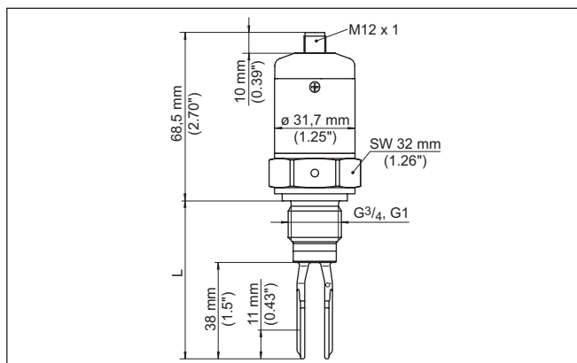
Abb. 31: VEGASWING S51 avec connecteur à fiches M12 x 1
