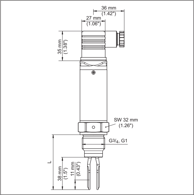
Abb. 44: VEGASWING S51 versión de alta temperatura con enchufe de válvula DIN 4400
