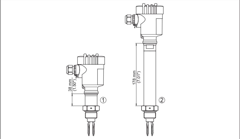
Fig. 19: Options 1)
