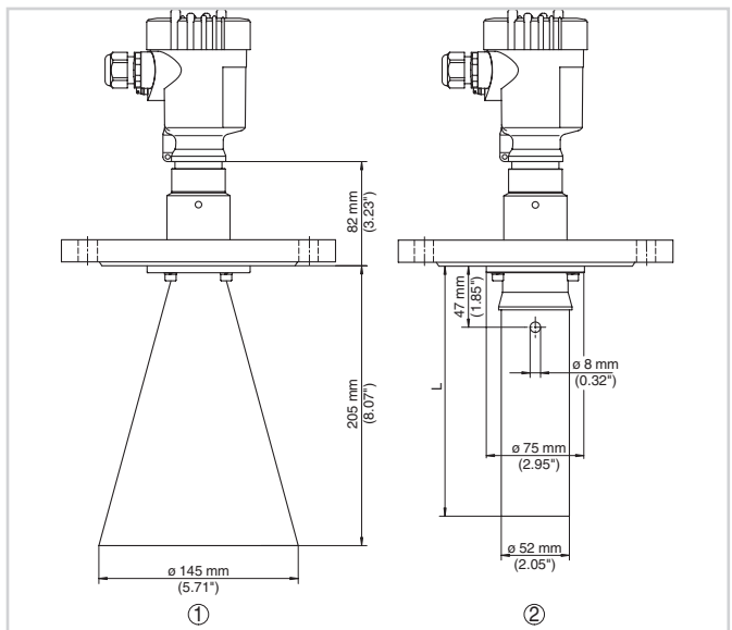
Dimensions VEGAPULS 66
