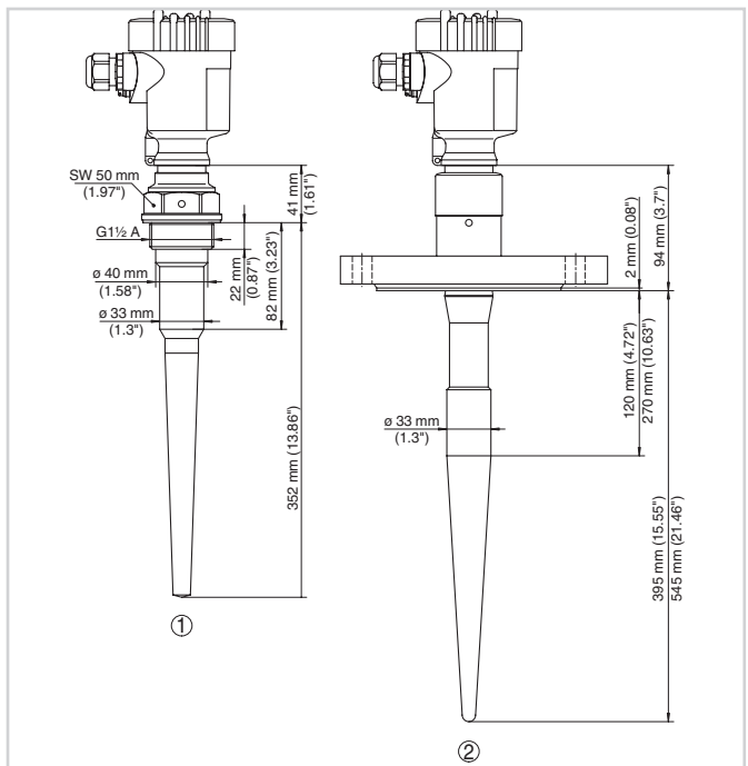
Dimensions VEGAPULS 65
