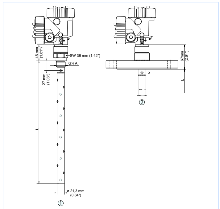
VEGAFLEX 65
