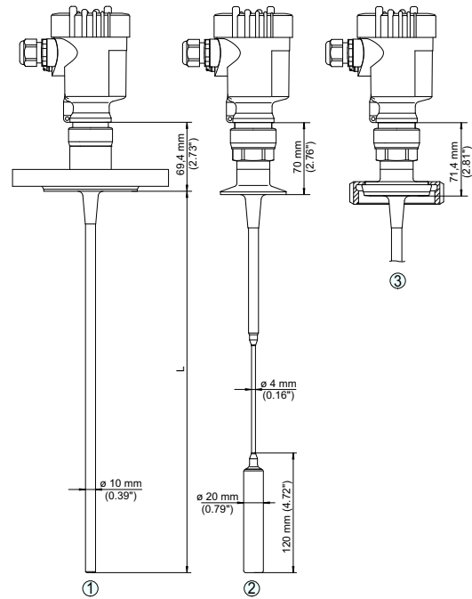
VEGAFLEX 63
