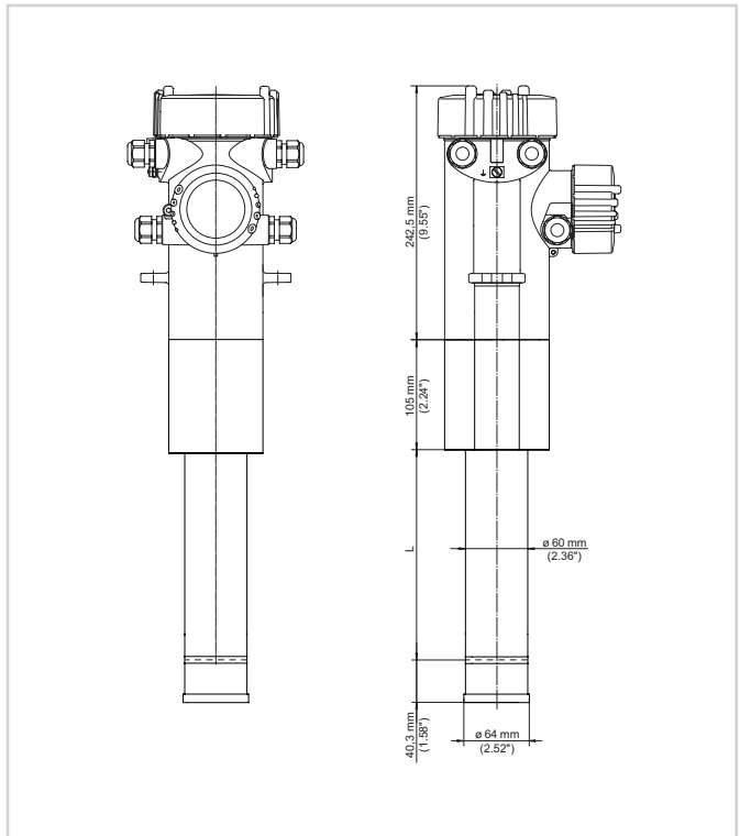
Dimensions FIBERTRAC 32
