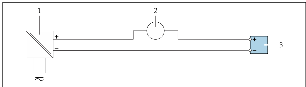
图 20 4...20 mA 电流输入的连接实例
