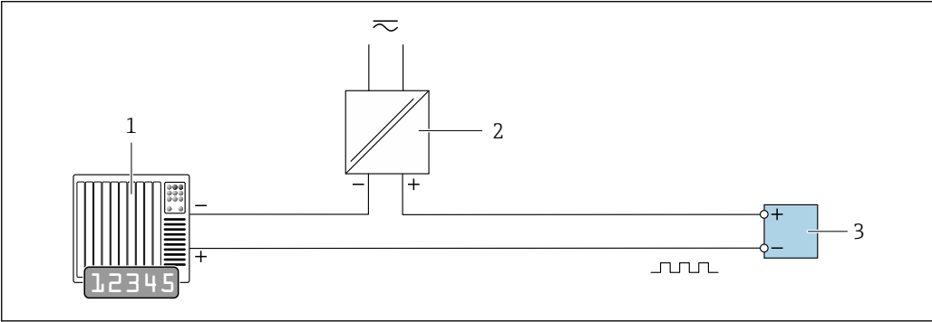
图 17 脉冲/频率输出(无源信号)的连接实例
