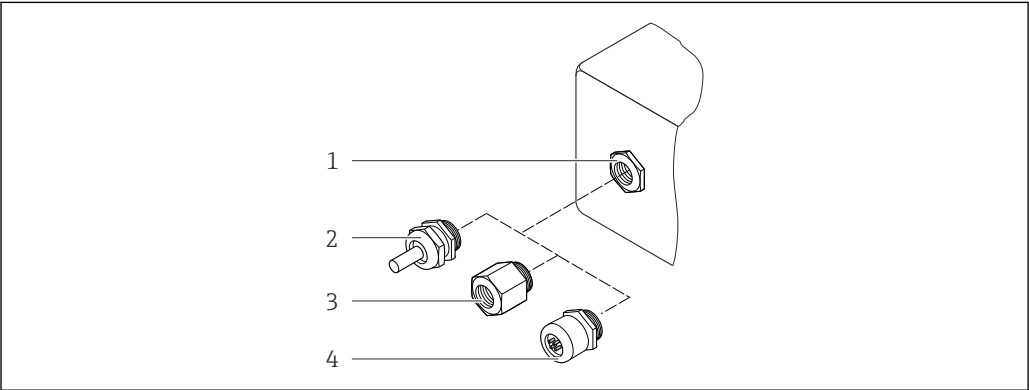
图 35 允许的电缆入口/缆塞
