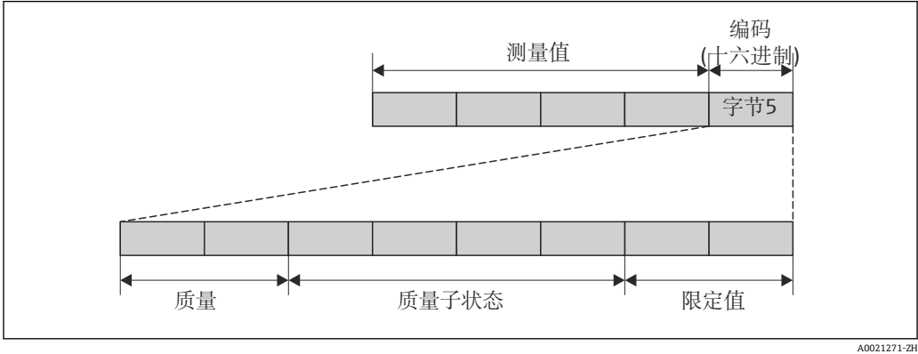
图 32 编码字节的结构
