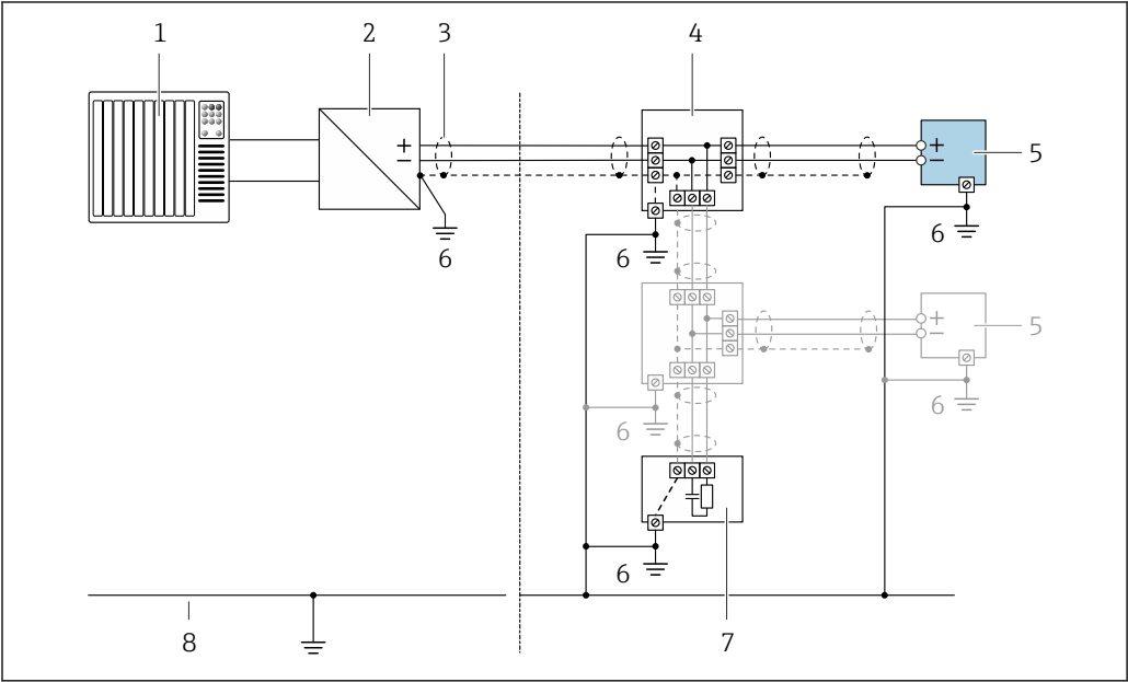
14 PROFIBUS PA 的连接实例
