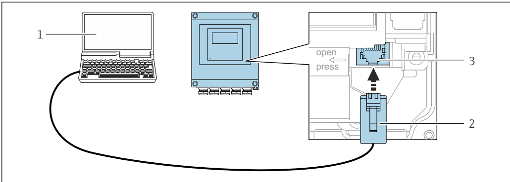
图 25 通过服务接口 (CDI-RJ45) 操作
