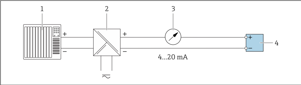
图 16 4...20 mA 无源电流输出的连接实例
