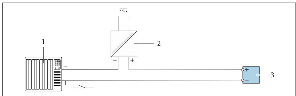
图 21 状态输入的连接实例
