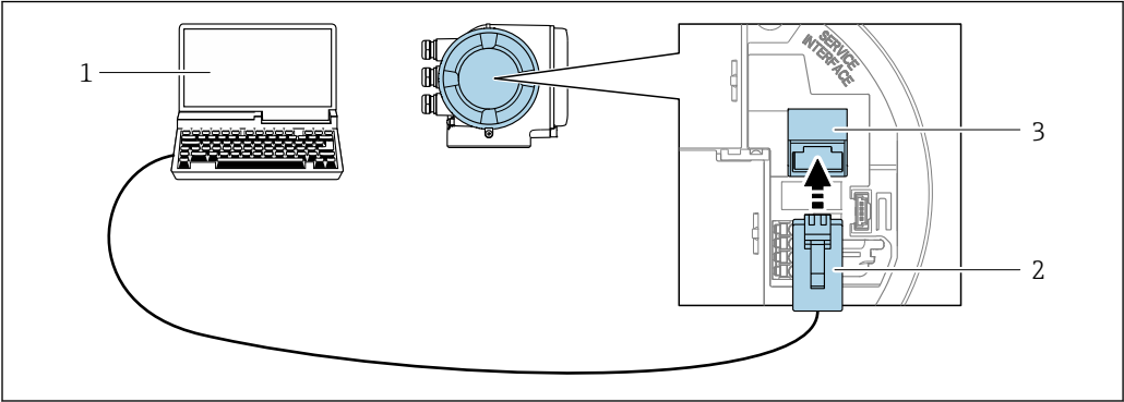
图 26 通过服务接口(CDI-RJ45)操作
