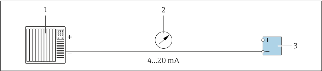
15 4...20 mA 有源电流输出的连接实例
