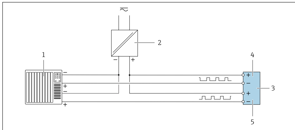
图 24 接线实例：双脉冲输出（无源信号）
