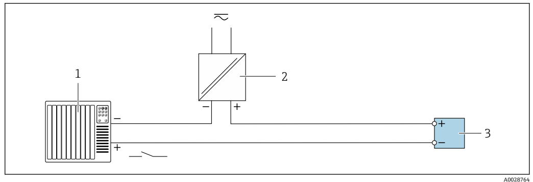
图 27 接线实例：状态输入
