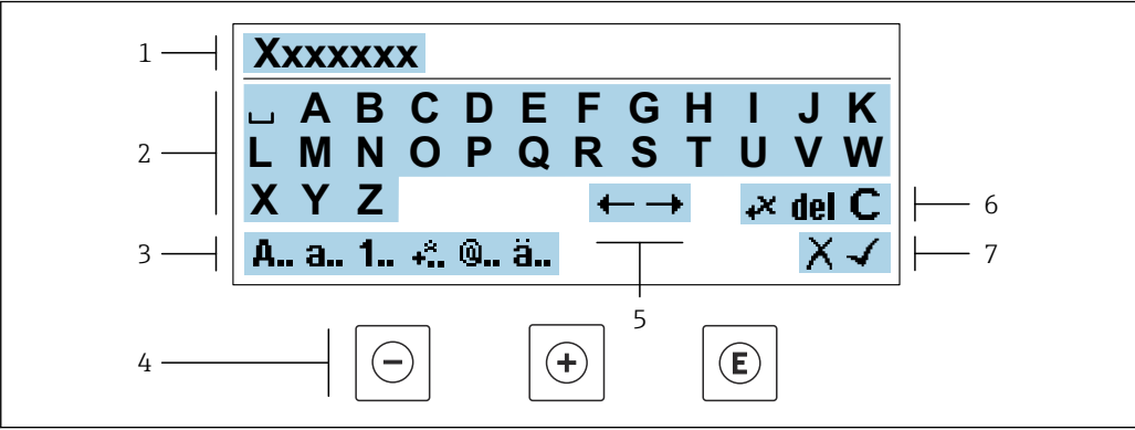
图 30 输入文本参数（例如设备位号）
