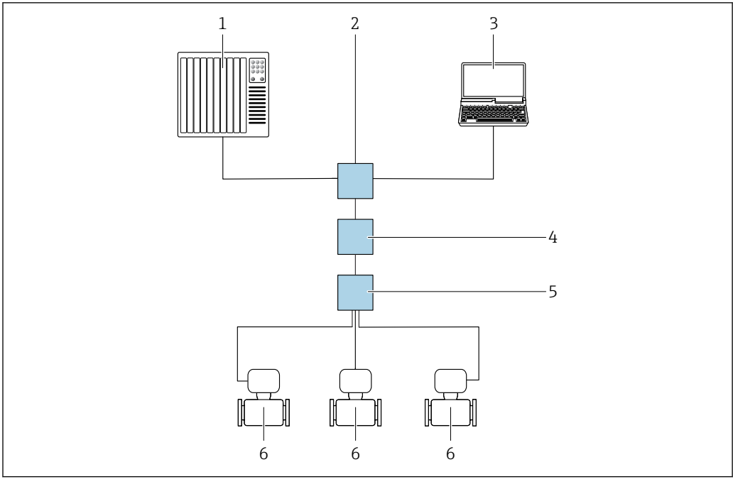
图 28 通过 Modbus TCP + Ethernet-APL 通信进行远程操作（有源信号）
