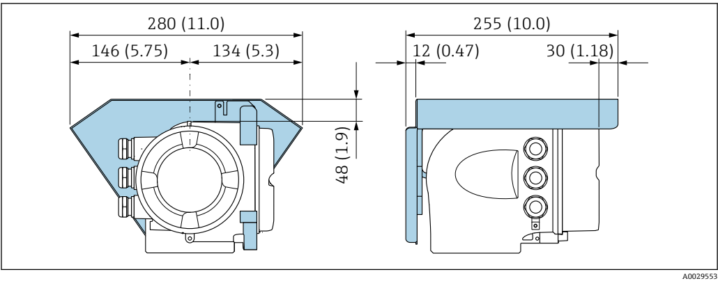
图 10 防护罩 (Proline 500) ; 单位: mm (in)
