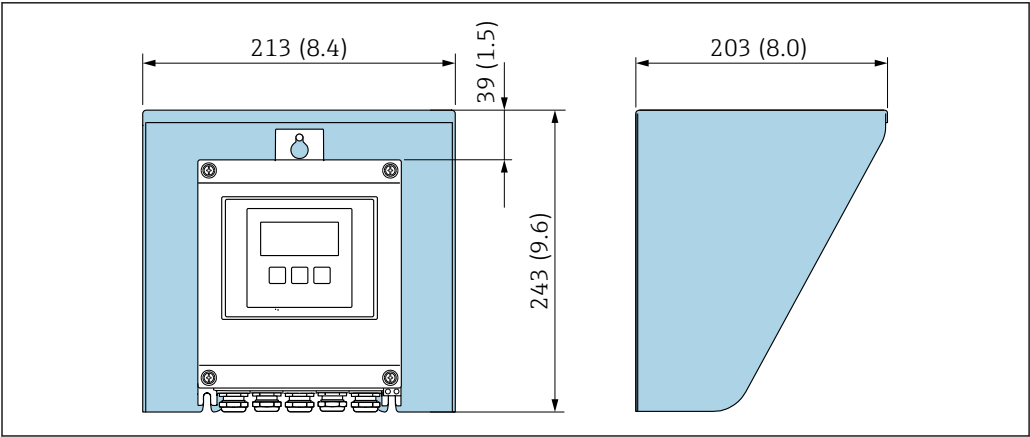
图 9 防护罩 (Proline 500 (数字式)) ; 单位: mm (in)
