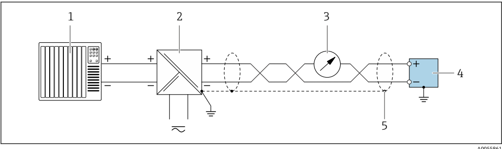
18 接线实例：4 ... 20 mA HART 电流输出（无源） 1 自动化系统，带 4 ... 20 mA HART 电流输入（例如 PLC） 2 电源 3 选配显示单元：注意最大负载 4 变送器，带 4 ... 20 mA HART 电流输出（无源） 5 电缆屏蔽层单端接地。如需确保安装符合 NAMUR NE 89 标准，电缆屏蔽层必须两端接地。
