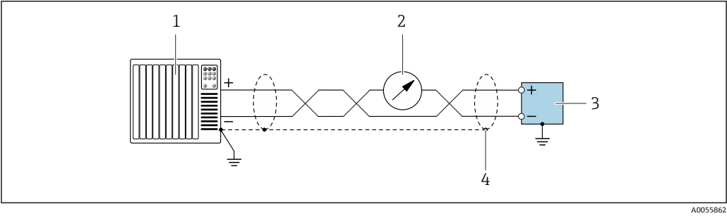
17 接线实例：4 ... 20 mA HART 电流输出（有源） 1 自动化系统，带 4 ... 20 mA 电流输入（例如 PLC） 2 选配显示单元：注意最大负载 3 变送器，带 4 ... 20 mA HART 电流输出（有源） 4 电缆屏蔽层单端接地。如需确保安装符合 NAMUR NE 89 标准，电缆屏蔽层必须两端接地。
