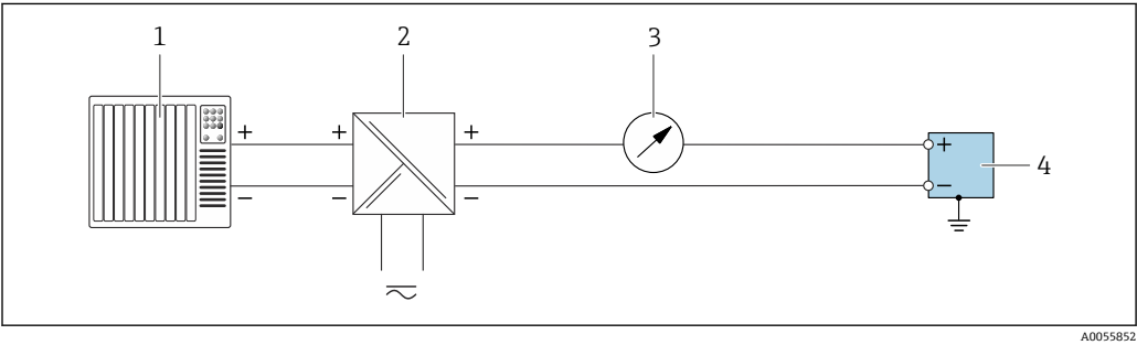
图 6 接线实例：4 ... 20 mA 电流输出（无源）
