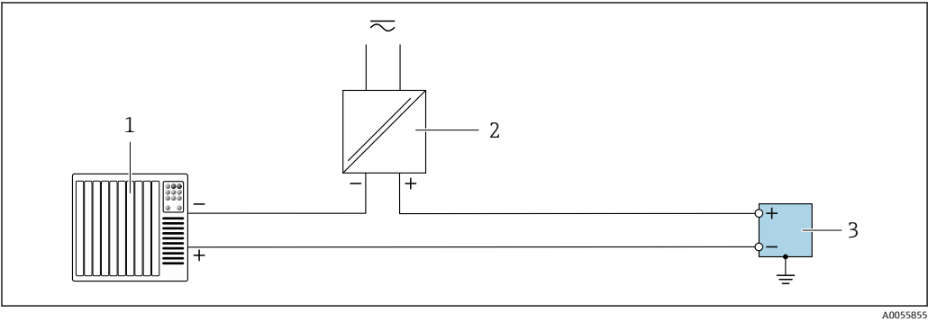
图 7 接线实例：脉冲输出/频率输出/开关量输出（无源）
