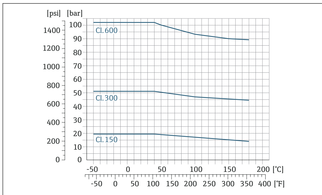
23 法兰材质: 1.4404 (316/316L)
