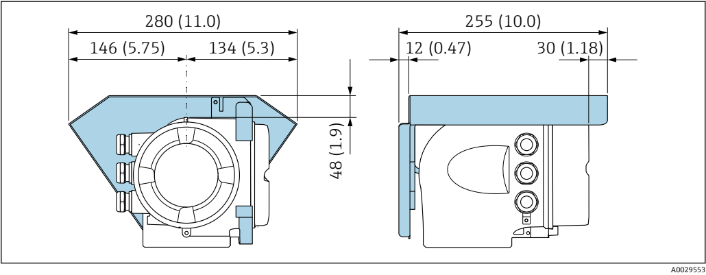
20 Proline 500 变送器的防护罩; 单位: mm (in)
