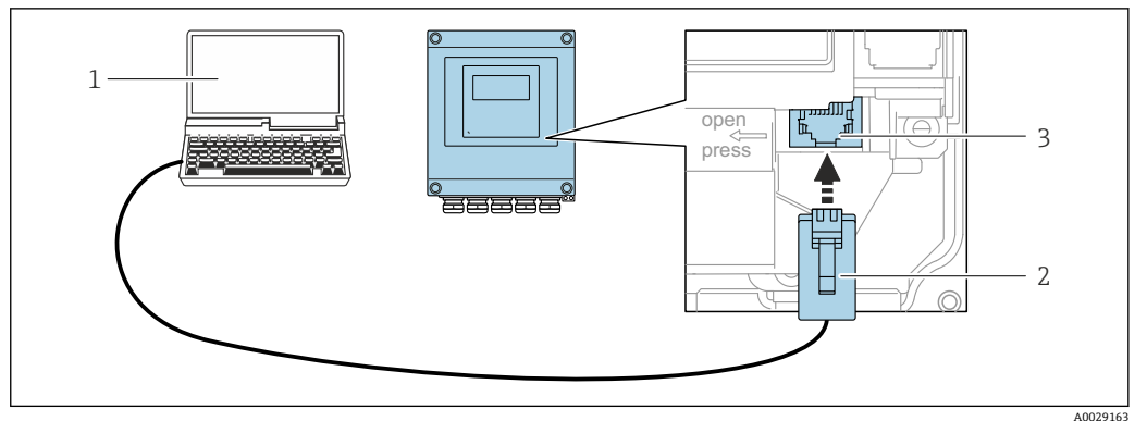
55 通过服务接口 (CDI-RJ45) 连接
