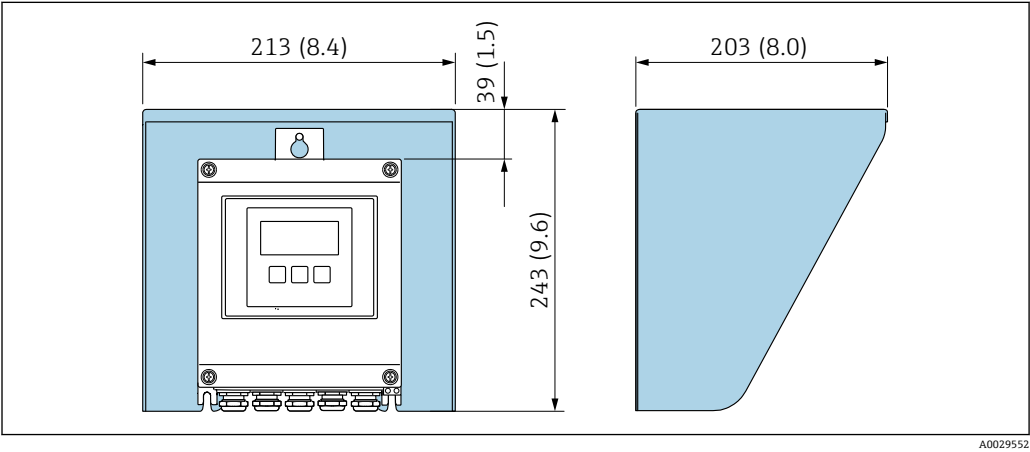
35 Proline 500（数字）变送器的防护罩；单位：mm (in)
