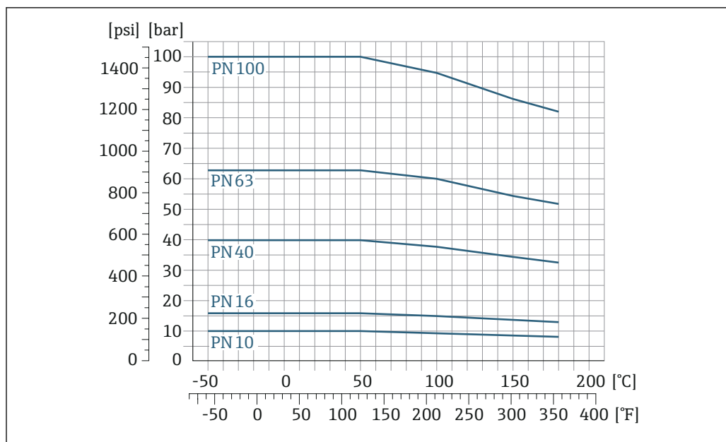
22 法兰材质: 1.4404 (316/316L)
