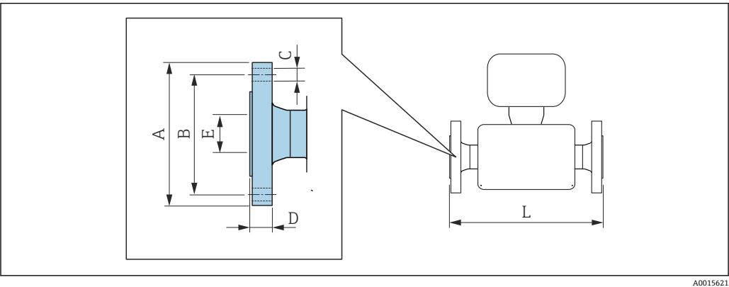
33 单位: mm (in)
