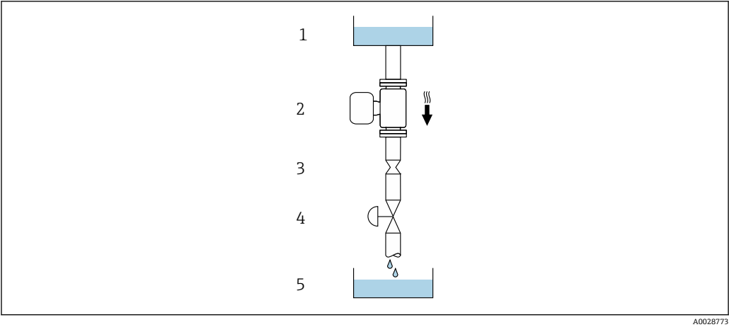
图 13 安装在竖直向下管道中（例如批处理应用）
