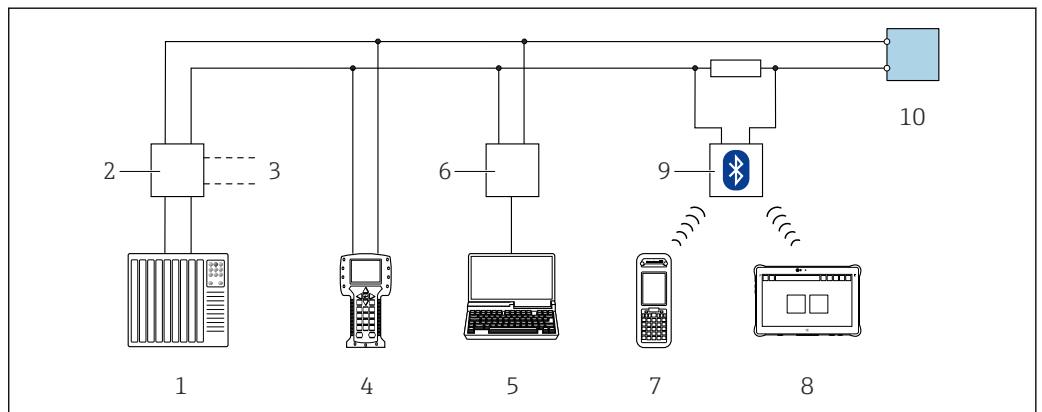
图 44 通过 HART 通信进行远程操作（无源信号）
