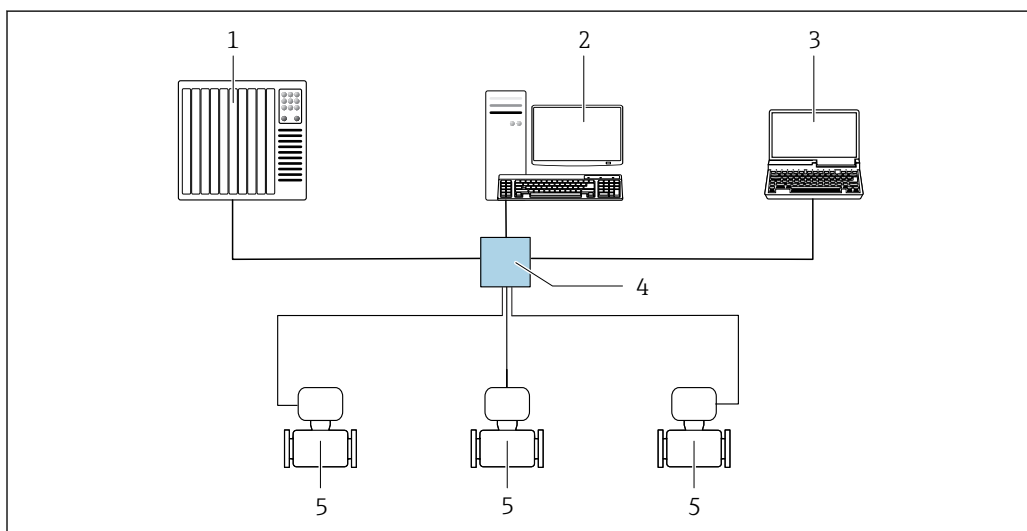
图 54 通过 Modbus TCP + Ethernet 进行远程操作 - 100 Mbit/s: 星形拓扑结构
