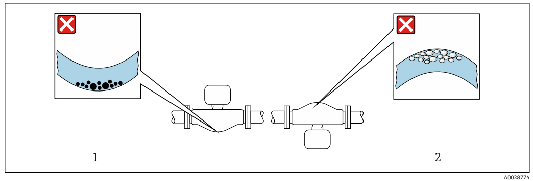
图 14 弯测量管传感器的安装方向
