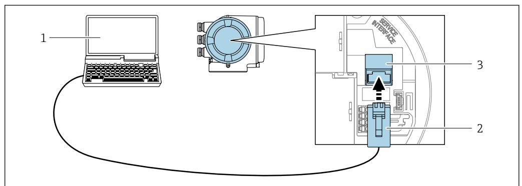
56 通过服务接口 (CDI-RJ45) 连接
