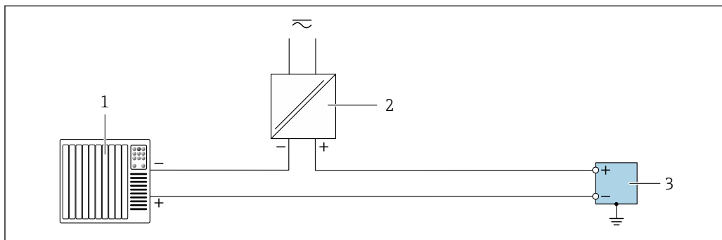
图 7 接线实例：继电器输出
