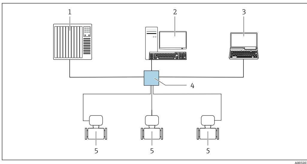
图 49 通过 EtherNet/IP 网络进行远程操作：星形拓扑结构
