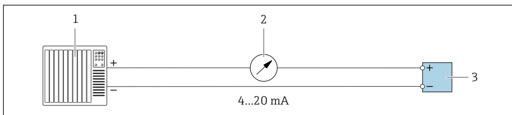
图 21 接线实例：4...20 mA 电流输出（有源信号）
