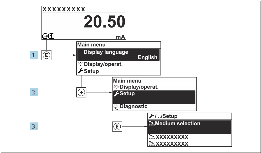
图 39 “设置”菜单菜单路径（现场显示单元）
