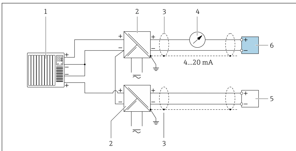
图 20 接线实例：HART 输入，公共端接负极（无源信号）
