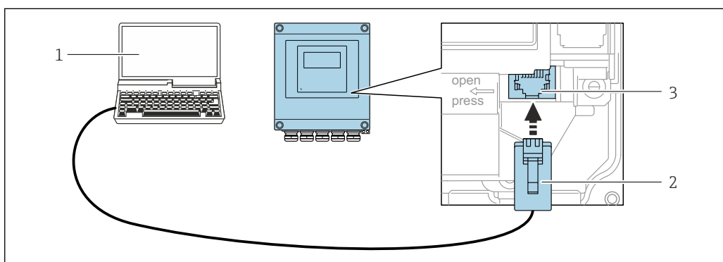
图 36 通过服务接口（CDI-RJ45）连接
