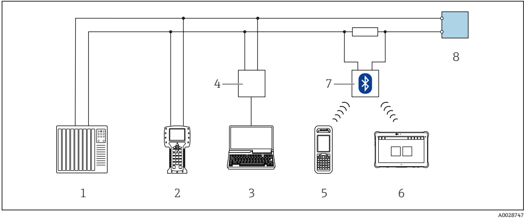
图 34 通过 HART 通信进行远程操作（有源信号）
