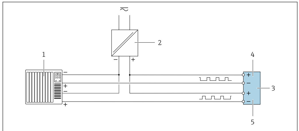
26 接线实例：双脉冲输出（无源信号）
