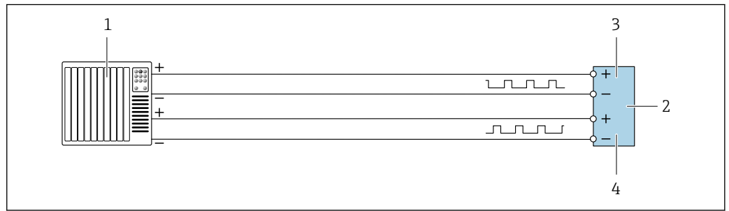
25 接线实例：双脉冲输出（有源信号）
