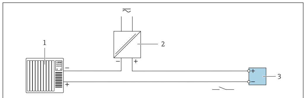
27 接线实例：继电器输出（无源信号）
