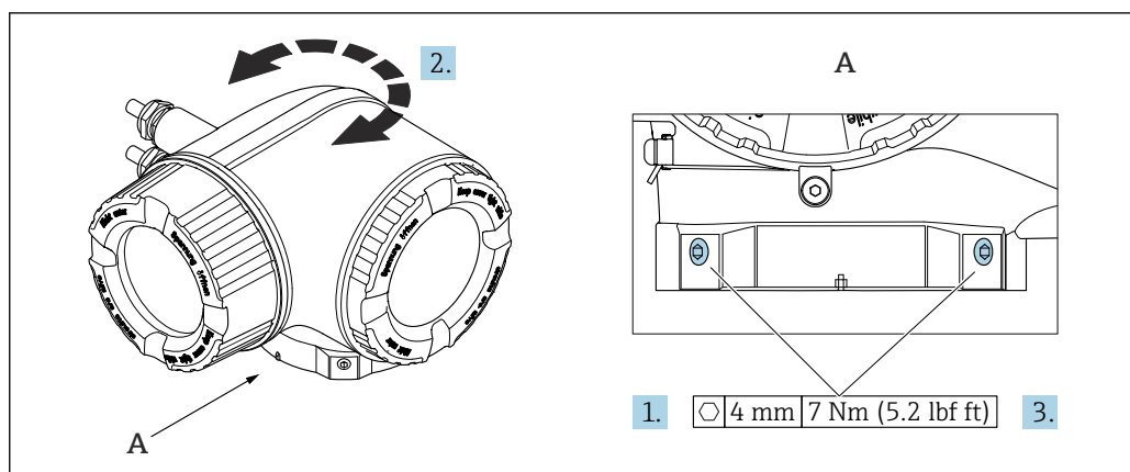
图 9 防爆型外壳
