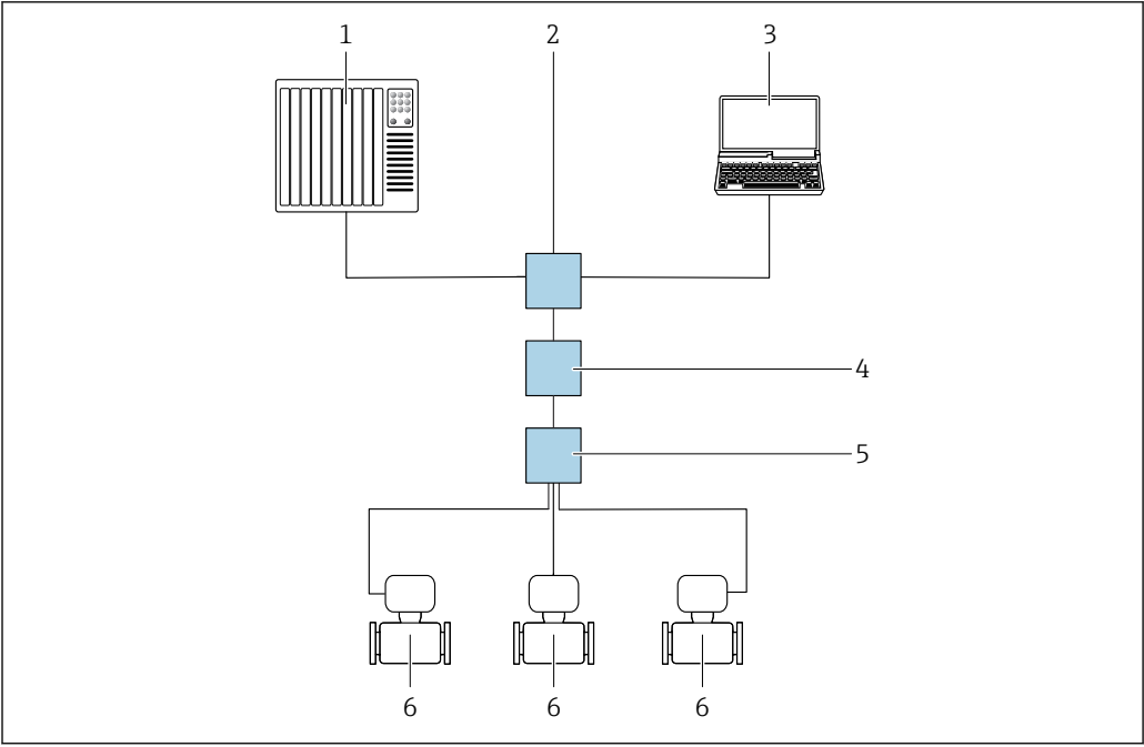
图 26 通过 Modbus TCP + Ethernet-APL 通信进行远程操作（有源信号）
