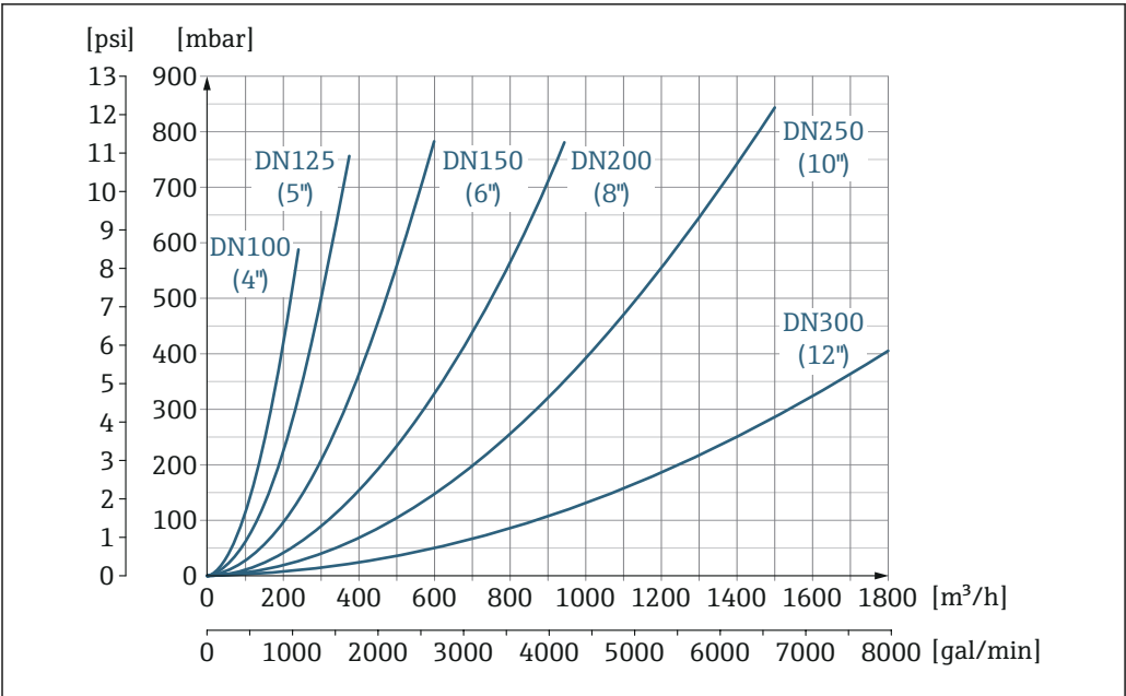
40 压损：适用口径 DN 100...300 (4...12"); 订购选项“设计”，选型代号 C “固定法兰，缩径测量管，无前后直管段长度要求”
