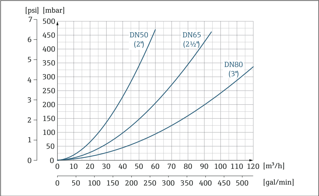
39 压损：适用口径 DN 50...80 (2...3"); 订购选项“设计”，选型代号 C “固定法兰，缩径测量管，无前后直管段长度要求”
