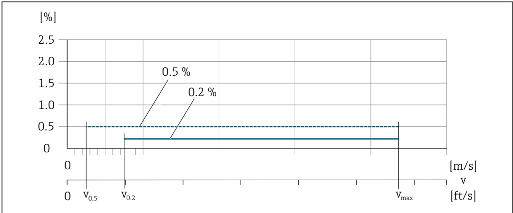
36 设计测量精度 (% o.r.)
