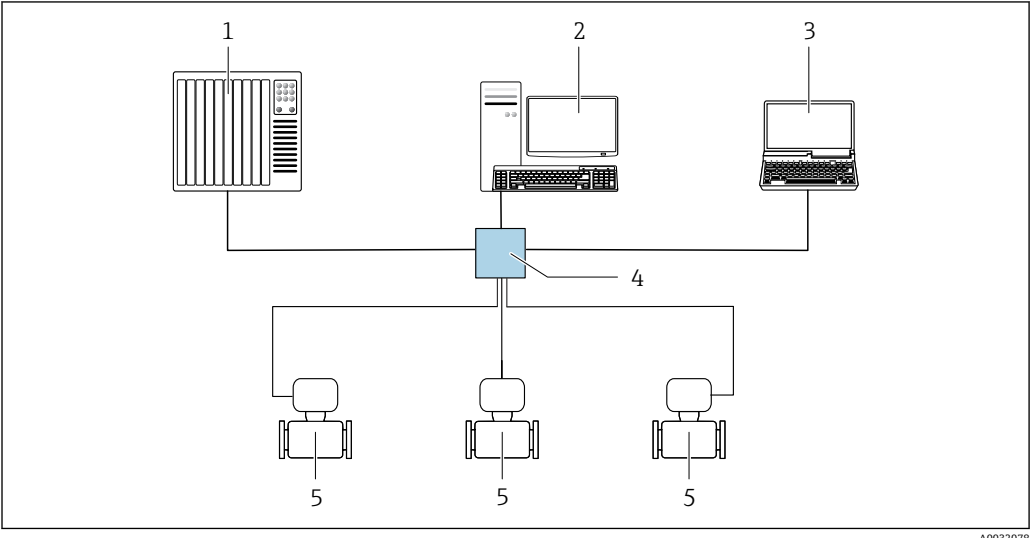
图 27 通过 Modbus TCP + Ethernet 进行远程操作 - 100 Mbit/s: 星形拓扑结构
