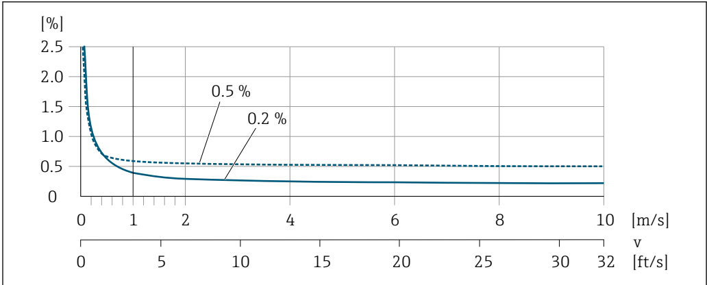
35 最大测量误差 (% o.r.)
