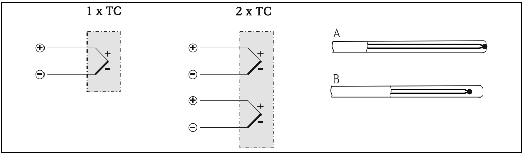
接线示意图
