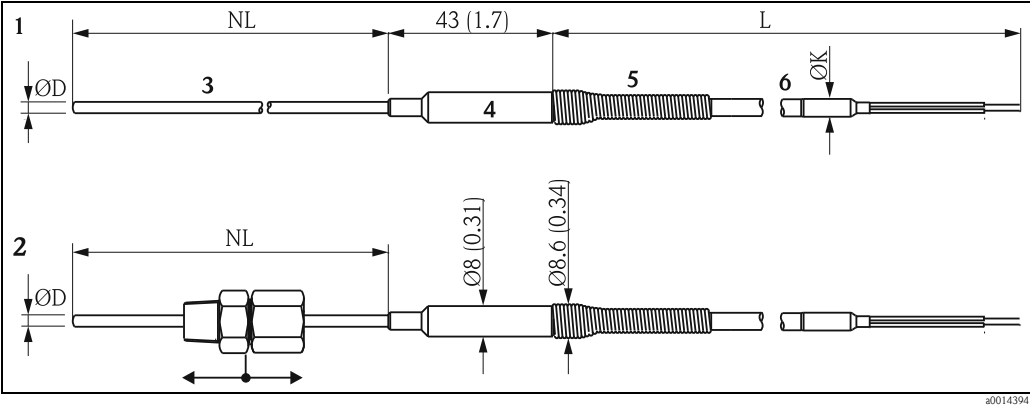
Omnigrad T TSC310 设计，单位：mm (in)
