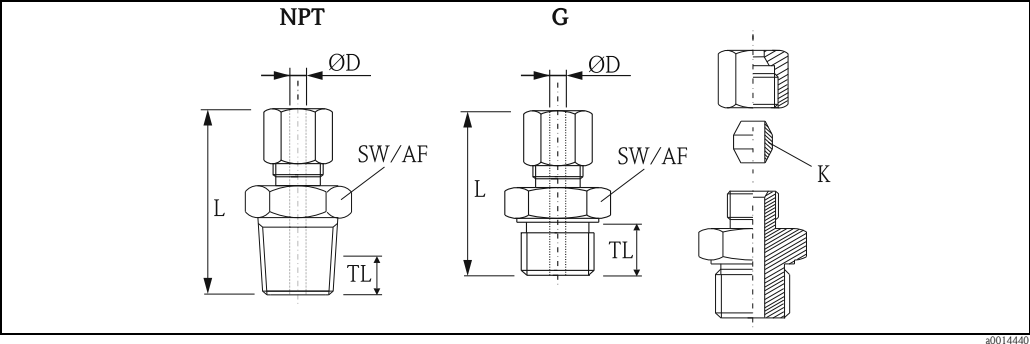
可调节卡套，带连接螺纹。单位：mm (in)
