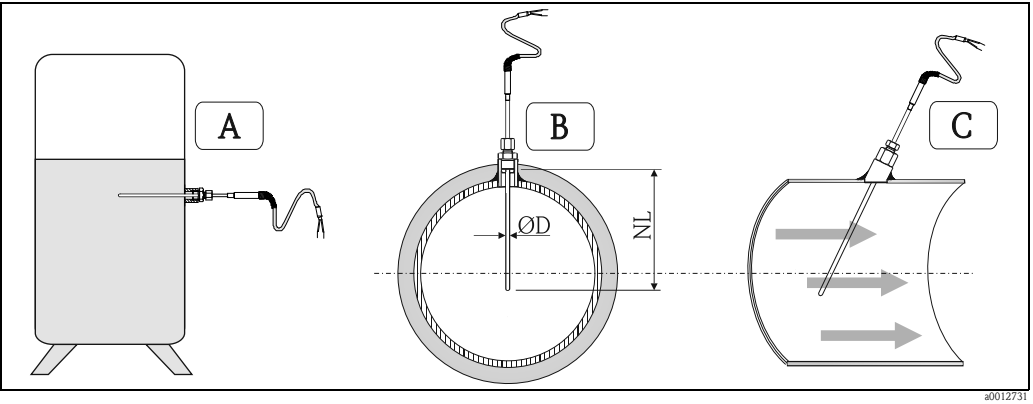
安装示意图 A: 安装在罐体中 B: 适用于小横截面积的管道，传感器末端应处于或稍微超出管道中心位置 (=NL) C: 倾斜安装
