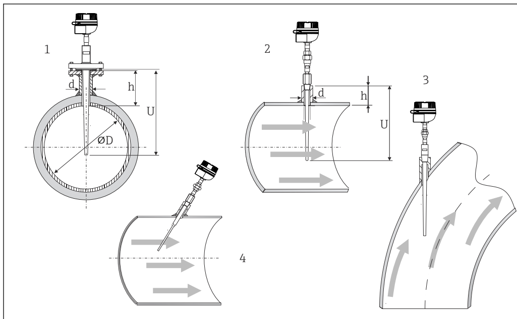
图 8 安装实例
