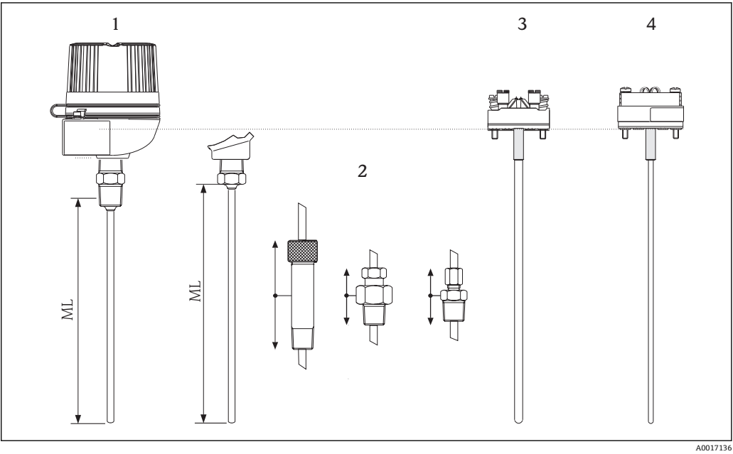
图 2 温度计的结构示意图 1 整套温度计，含接线盒和固定焊接螺纹 2 温度计，带可调节插入深度的过程连接 3 铠装芯子，已安装陶瓷接线端子(图例) 4 铠装芯子，已安装模块化变送器(图例) ML 插入深度
