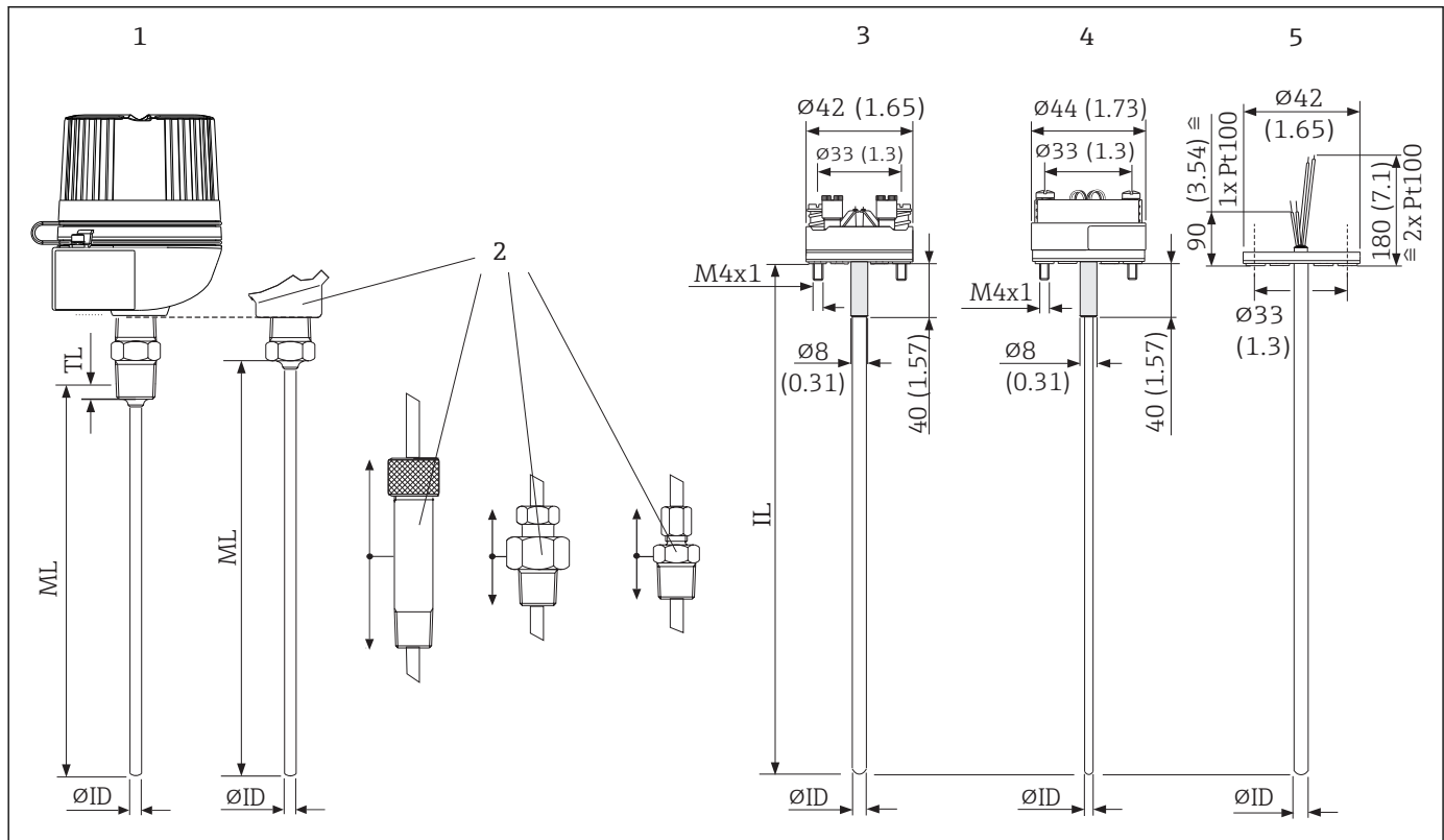
图 4 Omnigrad S TR65 和 TC65 的外形尺寸示意图
