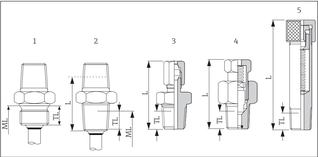
图 5 可选过程连接
