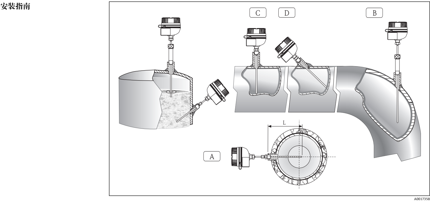
图 6 温度计的安装示意图 A、 竖直安装在小口径管道中，传感器末端应处于或略微超过管道中心位置(= L)。 C B、 倾斜安装 D
