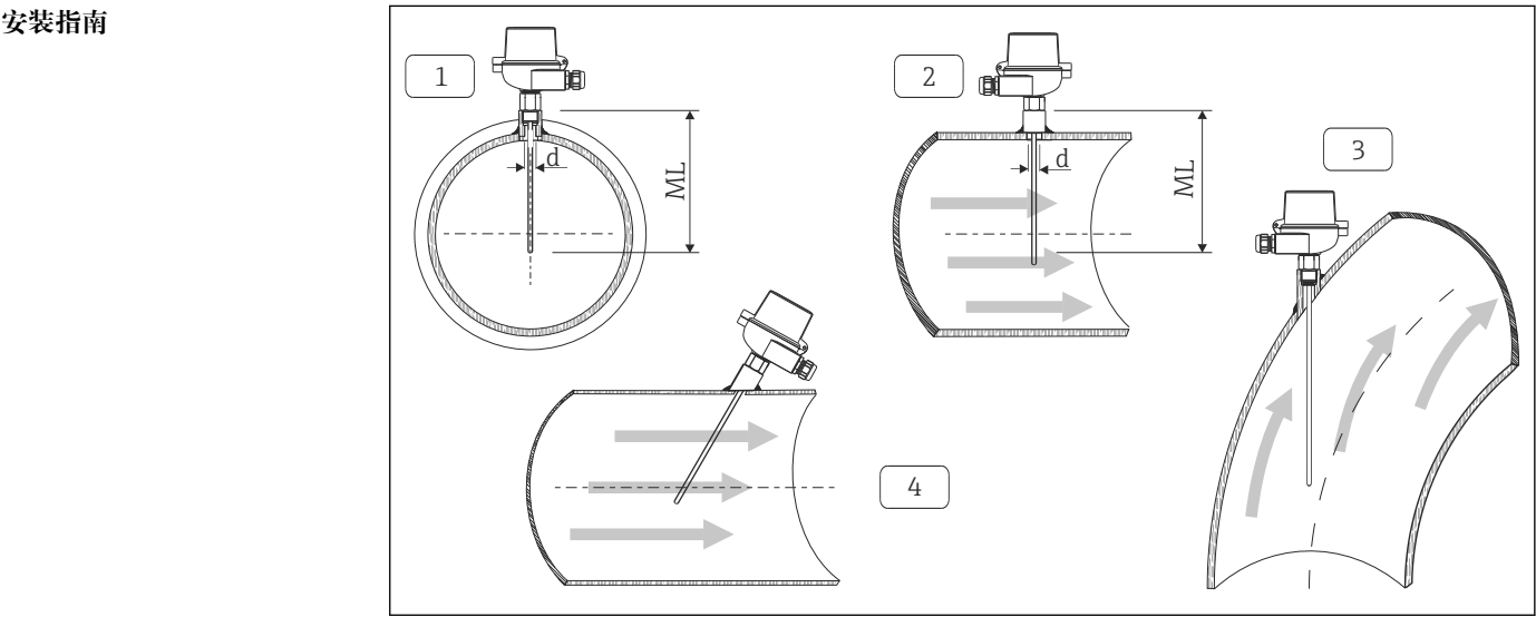
4 安装示意图
