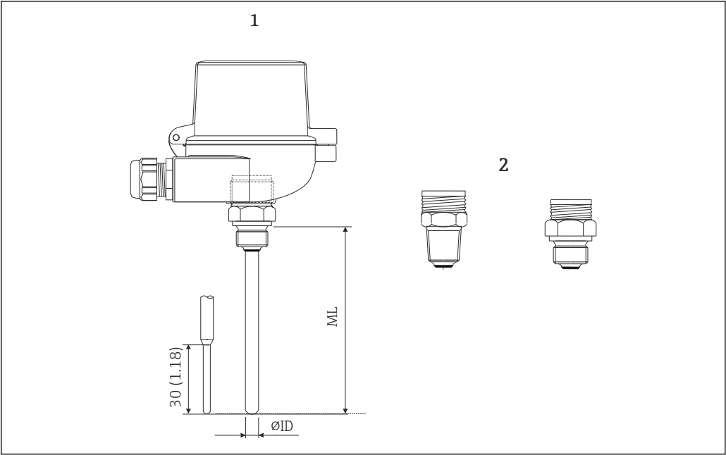
图 3 Omnigrad T TR25 外形尺寸示意图
