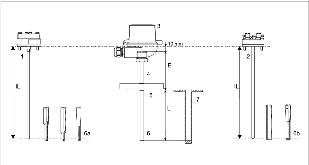
Omnigrad M TR13的设备结构
