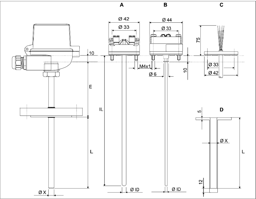
Omnigrad M TR13的机械尺寸
