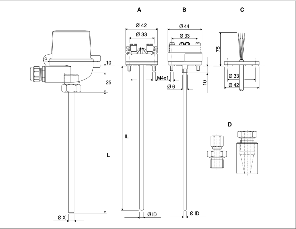
Omnigrad M TR12的机械尺寸
