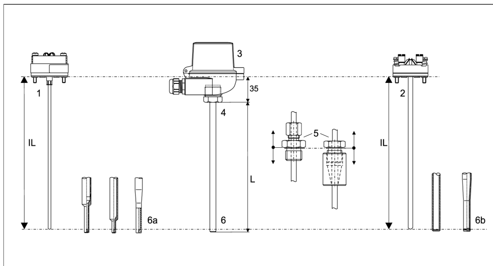
Omnigrad M TR12的设备结构
