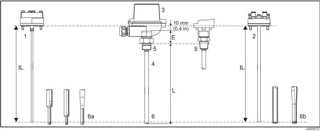
Omnigrad M TR11 的设备结构
