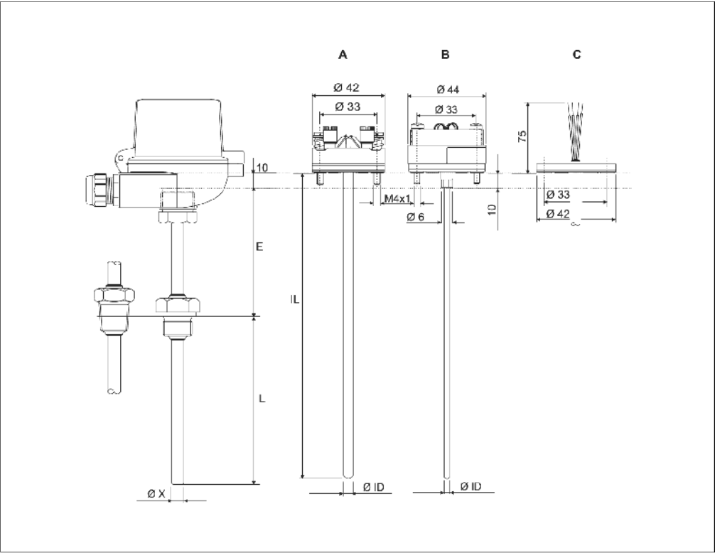
Omnigrad M TR10的机械尺寸
