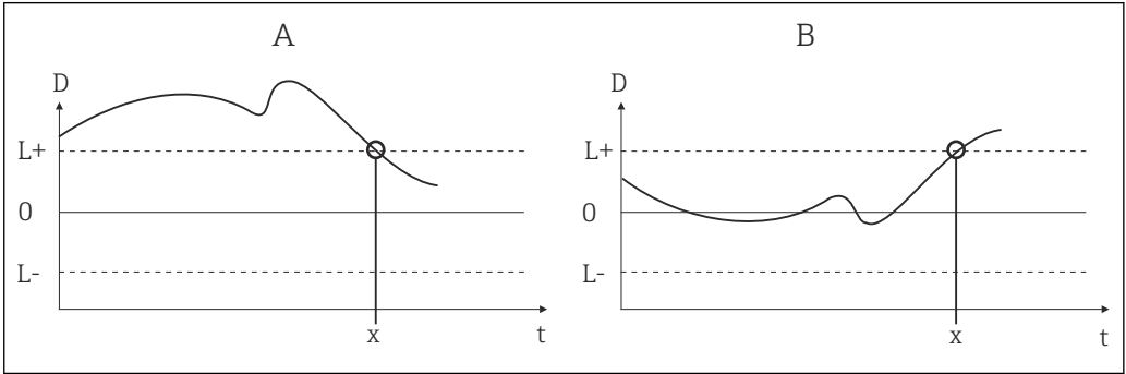
图 17 漂移检测 A “超量程下限”模式 B “超量程上限”模式 D 漂移 L+、上限 (+) 或下限 (-) 设定点 L- t 时间 x 错误 (故障) 或需要维护 (警告), 取决于设置
