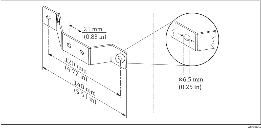
图 2 壁装架的外形尺寸（整套墙装套件可以作为附件订购）
