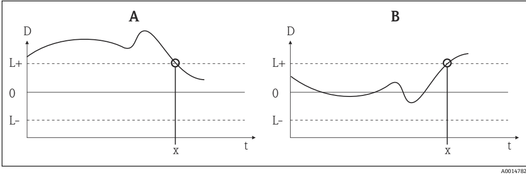
图 19 漂移/偏差模式 A 数值低于量程下限 B 数值高于量程上限 D 漂移 L+、上限 (+) 或下限 (-) 设定点 L- t 时间 x 诊断事件，发出状态信号
