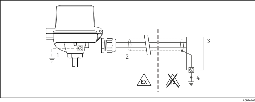
图 12 HART 通信电缆的单端屏蔽和接地连接
