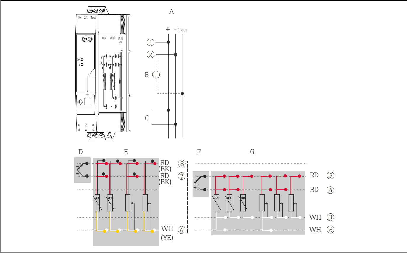
图 9 DIN 导轨式温度变送器的接线端子分配
