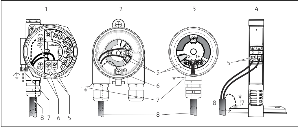
11 连接信号电缆和供电电缆
