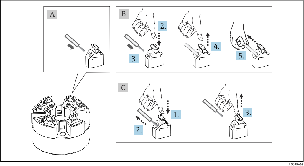
图 10 连接至直推式接线端子（以模块化温度变送器为例说明）
