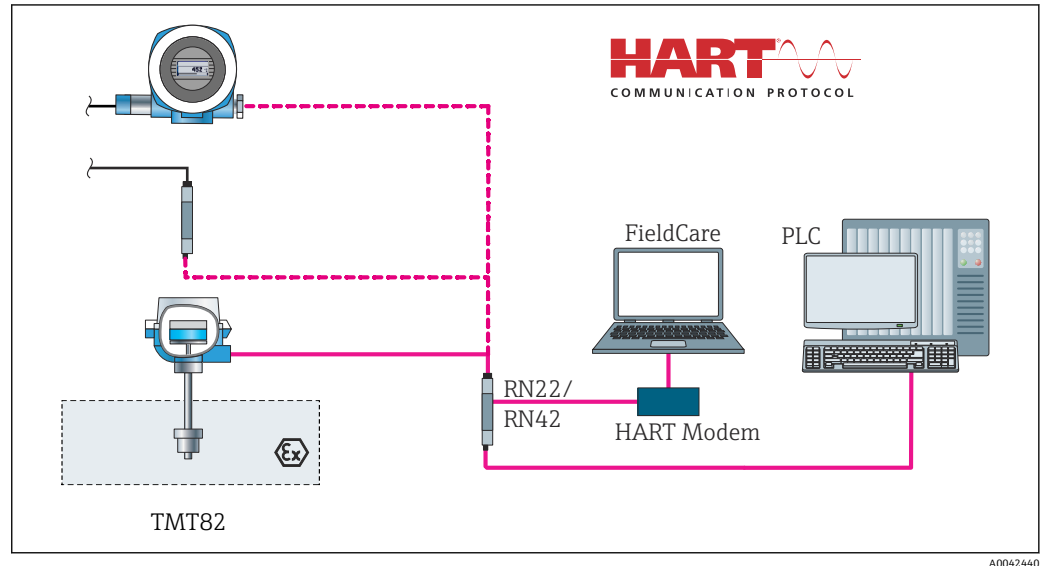
14 通过 HART 通信操作变送器
