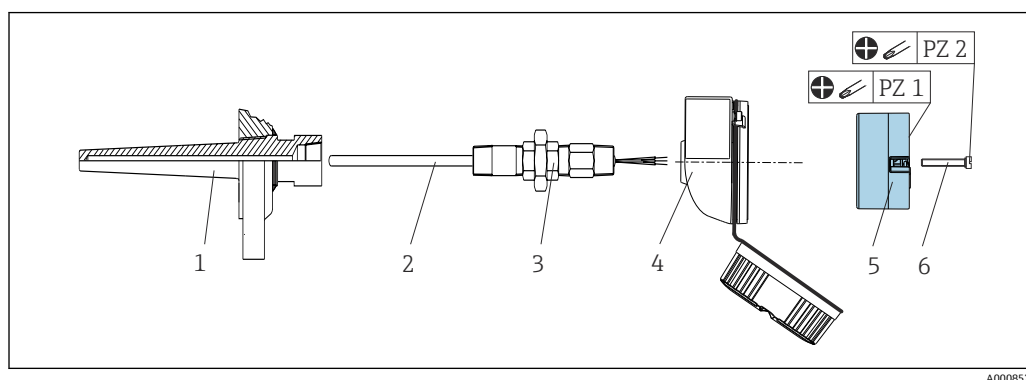
图 1 安装模块化温度变送器
