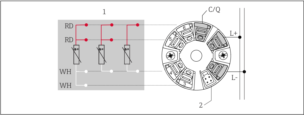
图 2 模块化温度变送器的接线端子分配
