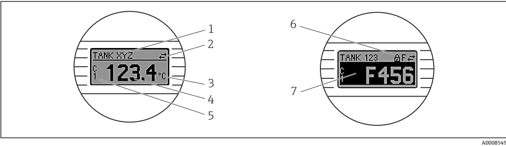
图 4 模块化温度变送器的液晶显示屏（选配）
