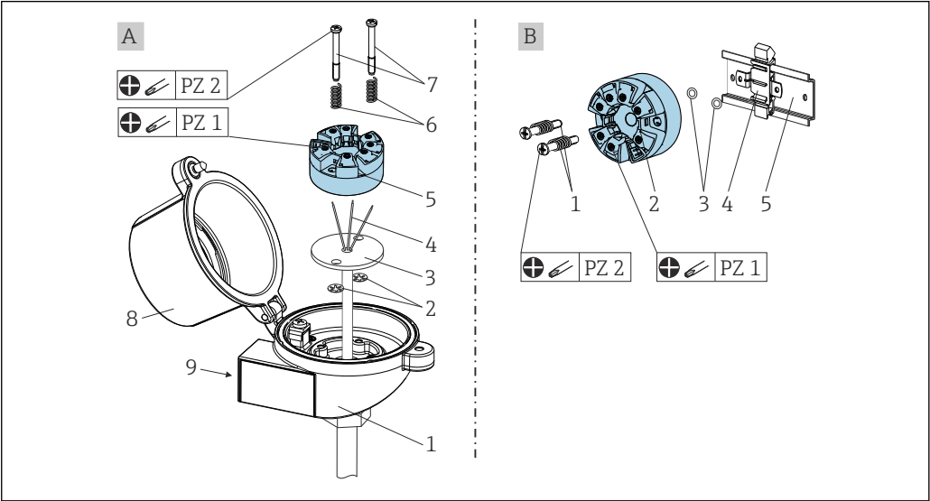
A 安装在符合 DIN EN 50446 标准的平面表头中，直接安装在带电缆入口的温度计芯子上（中心孔径：7 mm (0.28 in)） B 使用导轨夹安装在 DIN 导轨上，TH35 导轨符合 IEC 60715 标准
