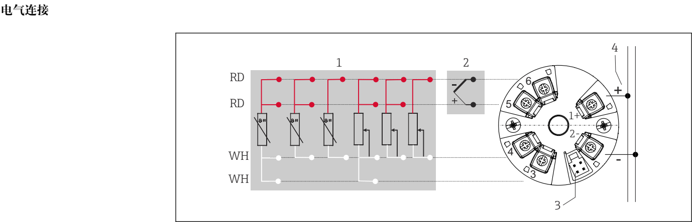
图 3 模块化变送器的接线端子分配示意图 1 传感器输入，热电阻 (RTD) 和电阻 (Ω) 信号，四线制、三线制和两线制连接 2 传感器输入，热电偶 (TC) 和电压 (mV) 信号 3 CDI 接口 4 总线端连接器和电源
