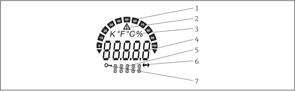
图 9 现场型变送器的液晶显示屏（背光显示，可插拔，每次旋转 90°）
