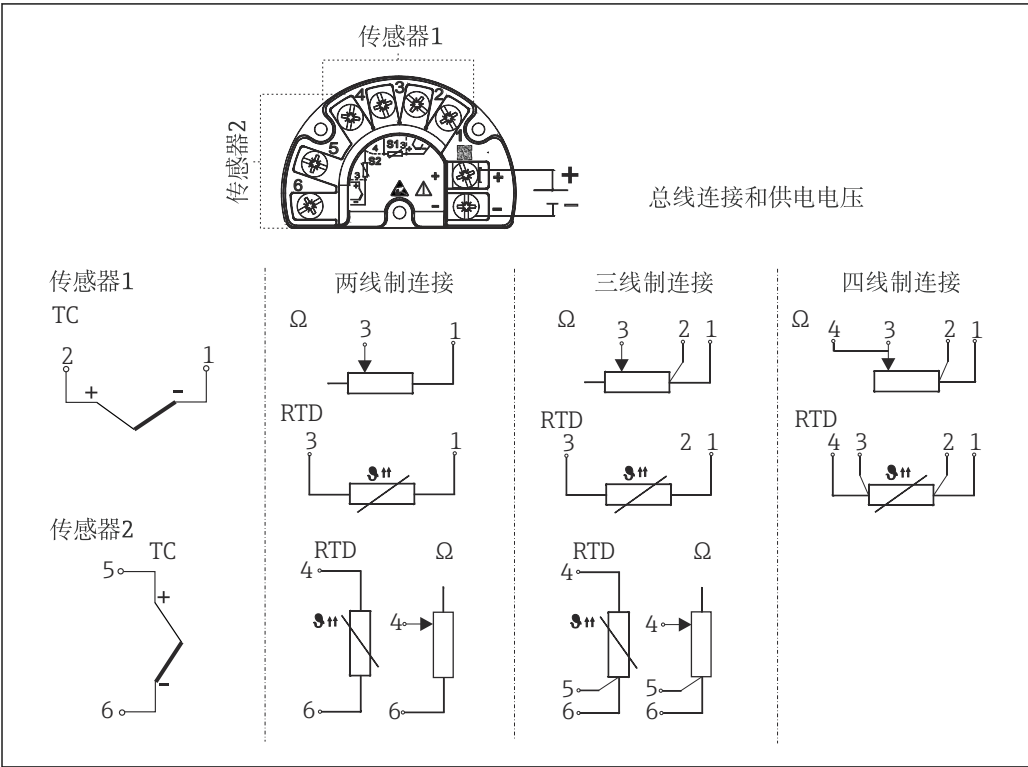
图 2 变送器接线
