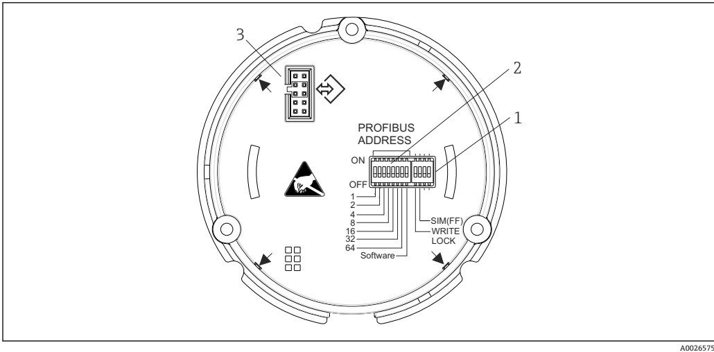
图 10 硬件设置，用于 FOUNDATION Fieldbus™和 PROFIBUS® PA 系统集成 1 DIP 开关，用于硬件写保护和仿真模式开关切换（FOUNDATION Fieldbus™仿真模式预设置） 2 DIP 开关，用于设置 PROFIBUS®设备地址 3 显示单元的电气连接
