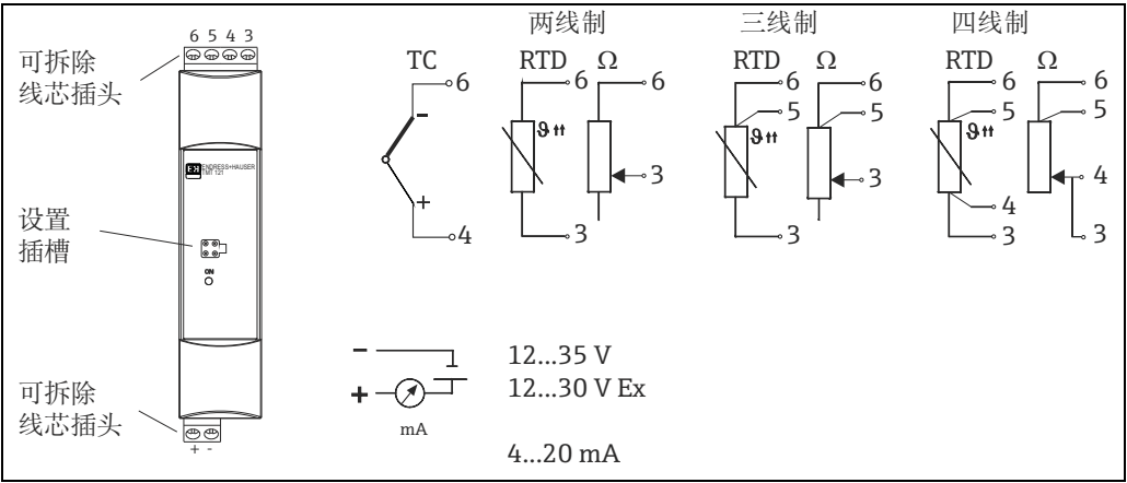
接线端子分配示意图
