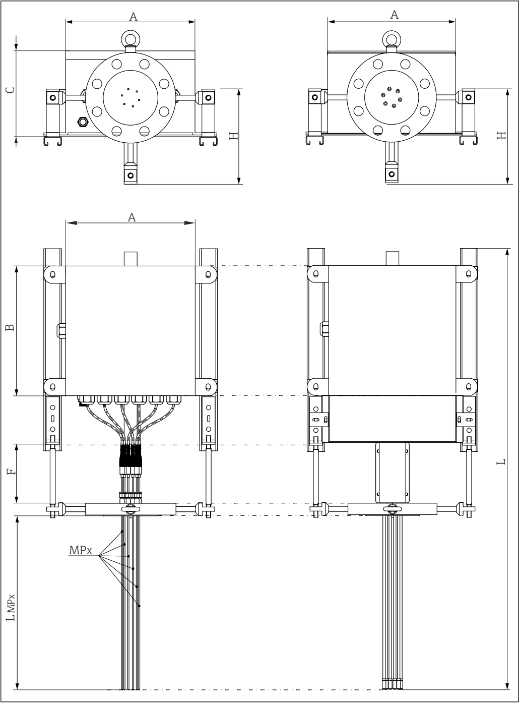
11 模块化多点温度计示意图，左图为带支撑板的型号，右图为带支撑板和外壳盖的型号。单位：mm (in)
