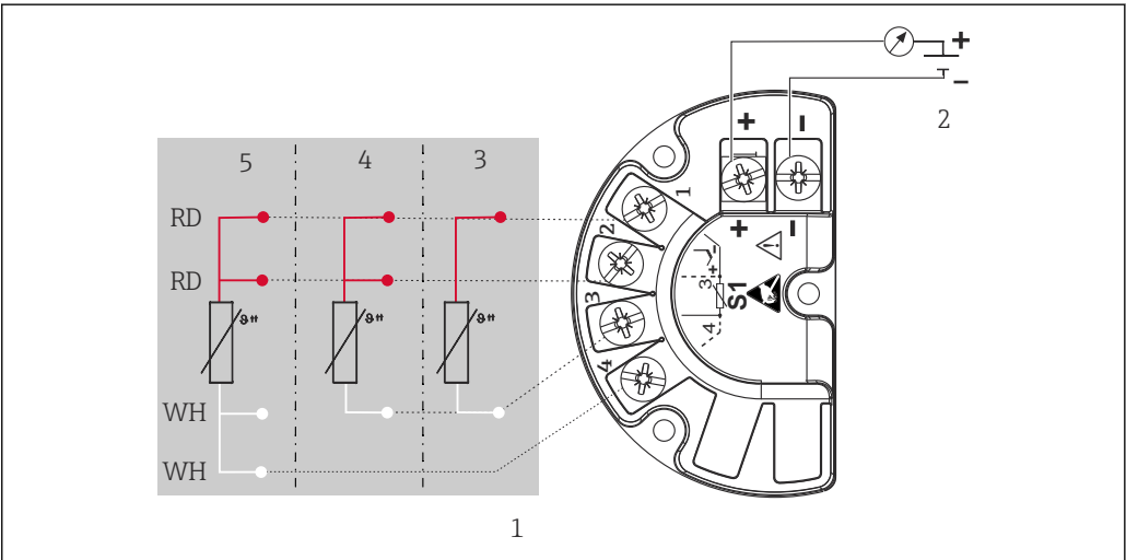
图 7 TMT142B (单输入通道)
