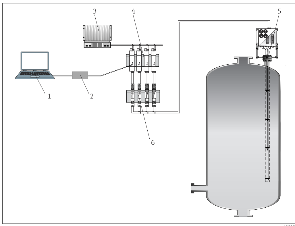
图 1 反应罐应用实例：多点温度计安装在现场提供的保护套管中，提供四个温度测量点，分体式接线箱中安装有四台变送器或四个端子接线排。
