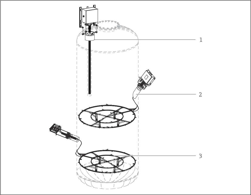
图 9 安装示意图：安装方向不受限制
