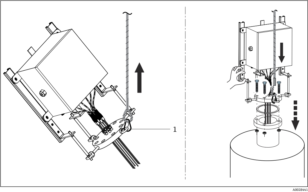
10 通过法兰连接将多点温度计安装在反应器的安装短管上
