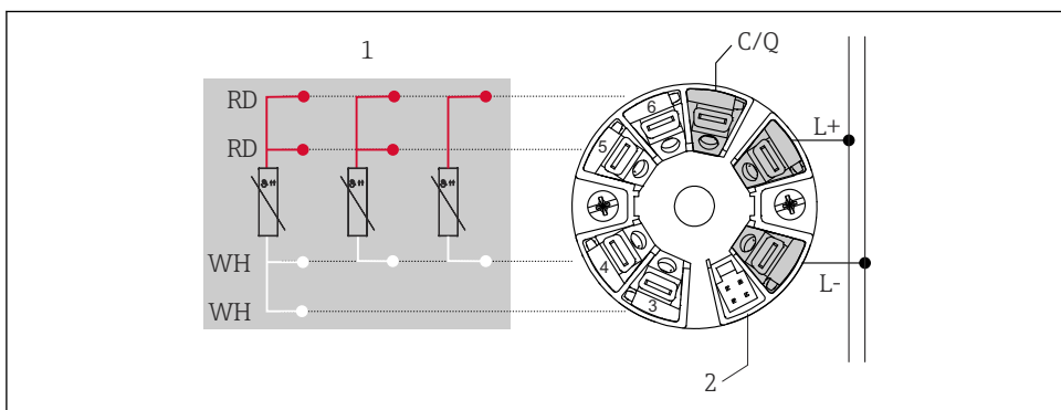
6 iTEMP TMT36 模块化温度变送器（单路传感器输入）
