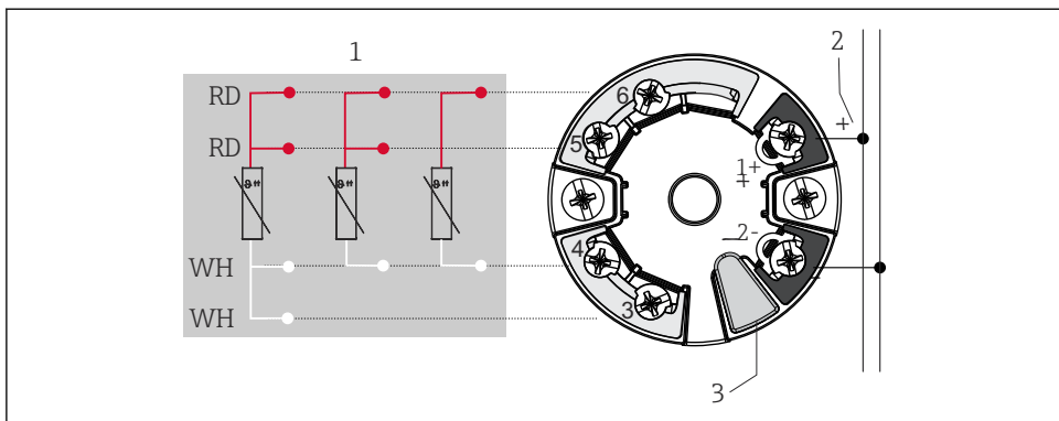
5 iTEMP TMT7x 或 iTEMP MT31 模块化温度变送器（单路传感器输入）
