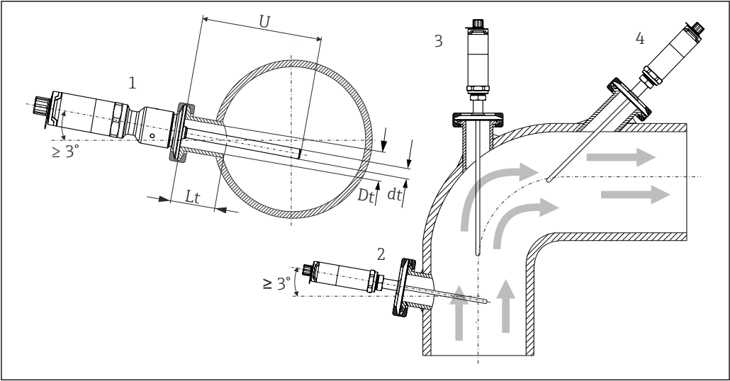
图 3 在过程中的允许安装位置
