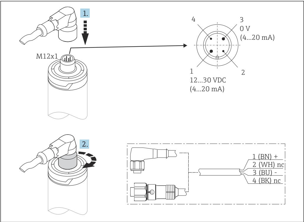
图 6 M12x1 电缆插头和设备连接插座的引脚分配
