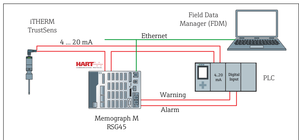
图 5 iTHERM TrustSens 连接至 4 ... 20 mA/RSG45 的 HART 输入。此外，4 ... 20 mA 信号也可以环路连接至一个 PLC，用于过程控制。RSG45 评估设备状态（测量值状态）并在发生警告/错误时通过继电器输出或现场总线（选装）输出一条信息。可以对 iTHERM TrustSens 进行配置和调试，例如，使用“FieldCare”PC 软件工具并利用以太网至 HART 的通信通过 RSG45 的以太网端口完成。
