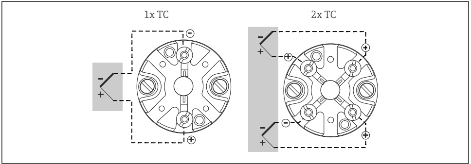
3 已安装的热电偶陶瓷端子接线块。
