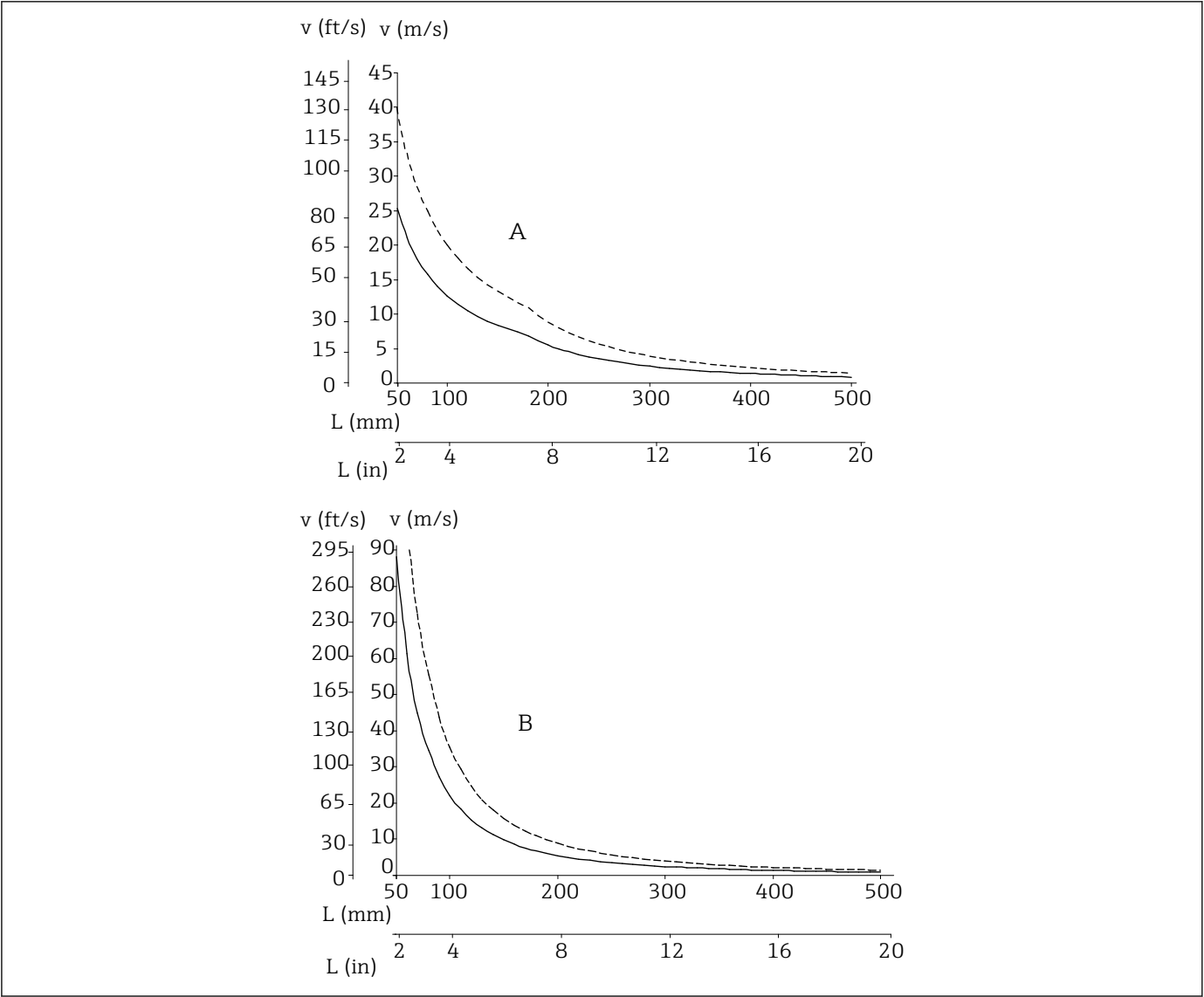
图 9 最大允许流速：9 mm (0.35 in)保护套管 (——) 或 12 mm (0.47 in)保护套管 (-----) A 水：T = 50 °C (122 °F) B 过热蒸汽：T = 400 °C (752 °F) L 插深 v 流速
