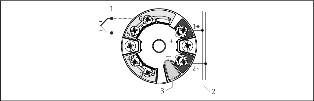
图 7 iTEMP TMT7x 或 iTEMPT MT31 模块化温度变送器（单路传感器输入）
