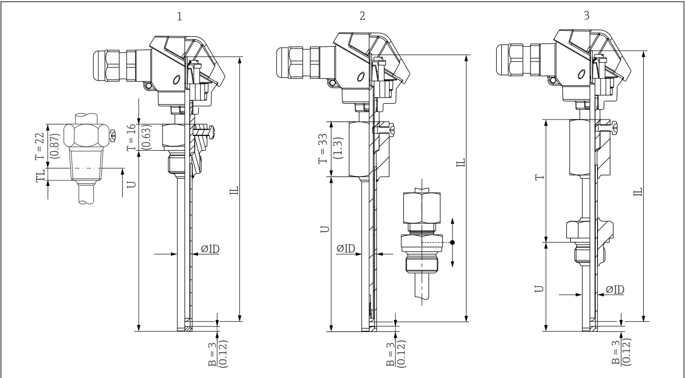
11 温度计，带 Mignon 表头
