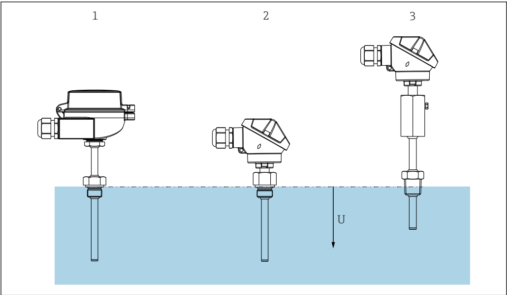
图 2 不同配置的温度计
