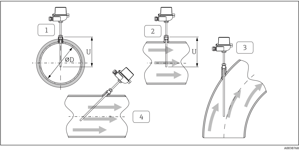
图 8 安装实例
